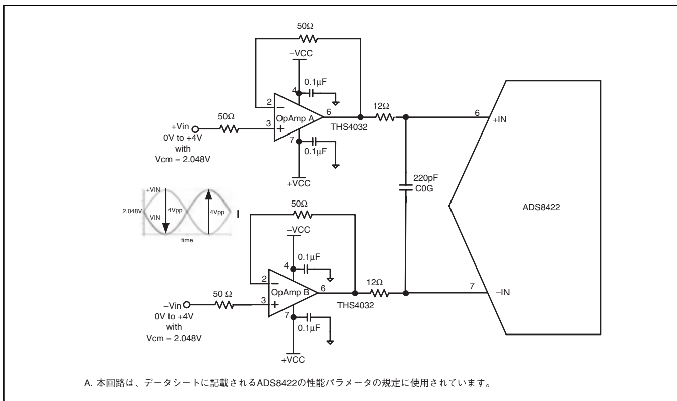
図32. 入力が2.048Vの同相電圧に乗る完全差動信号時の駆動回路
