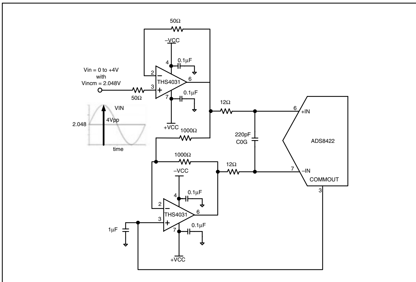
図31. 入力がシングルエンドのユニポーラ信号で2.048V同相電圧時のシングルエンド駆動回路
