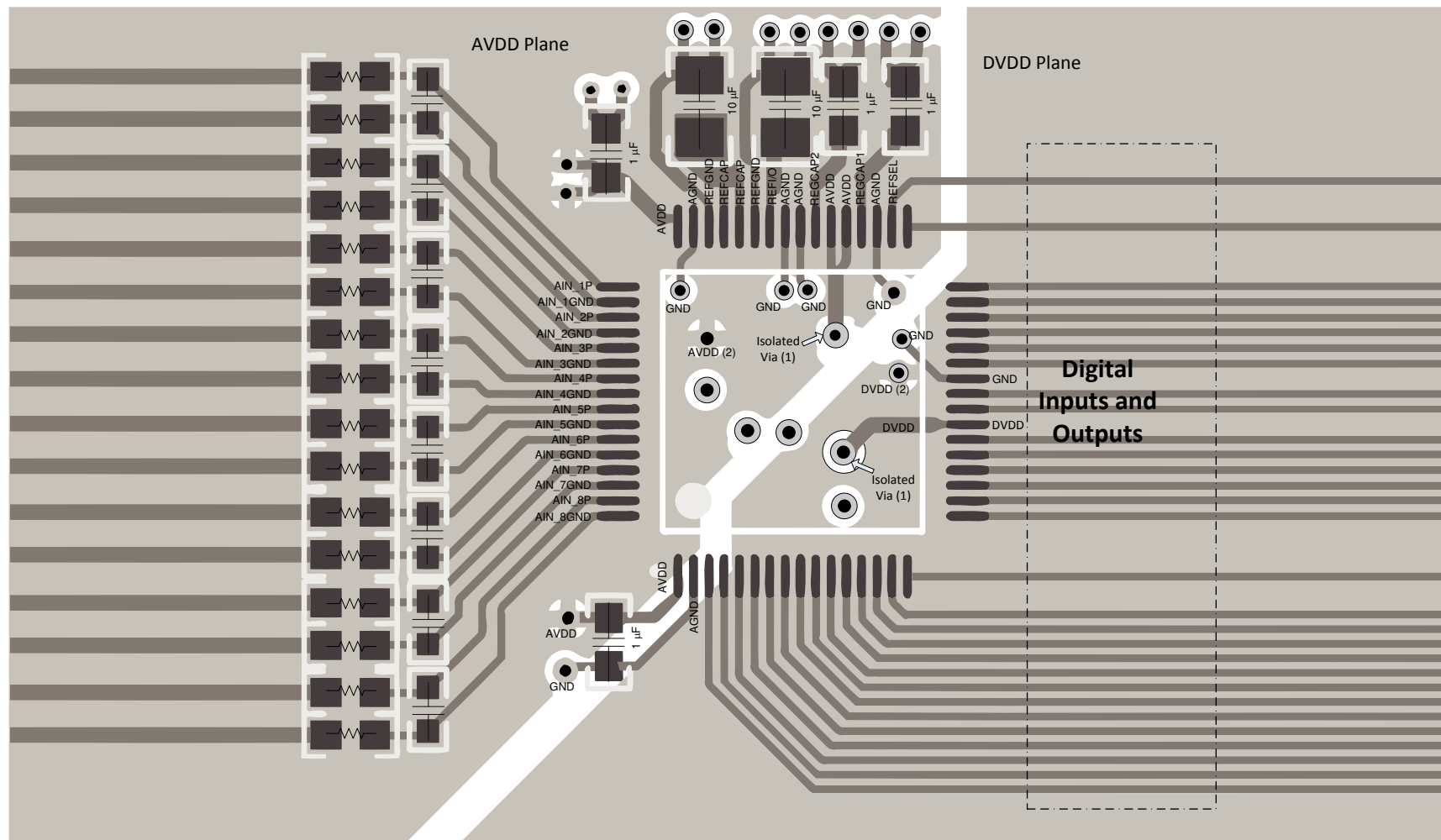
☒ 8-6. Top Layer Layout
