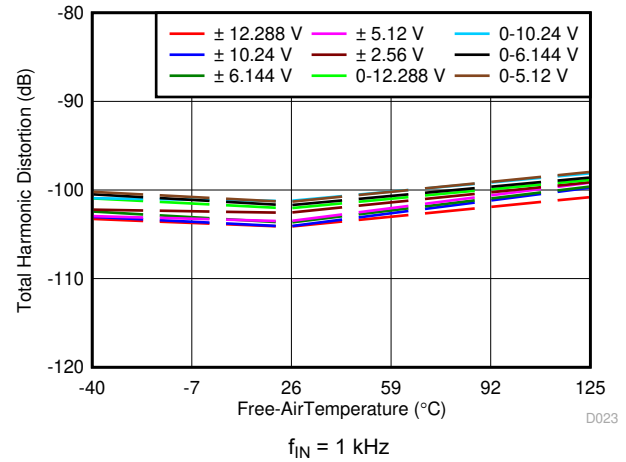
图 6-40. THD vs Temperature
