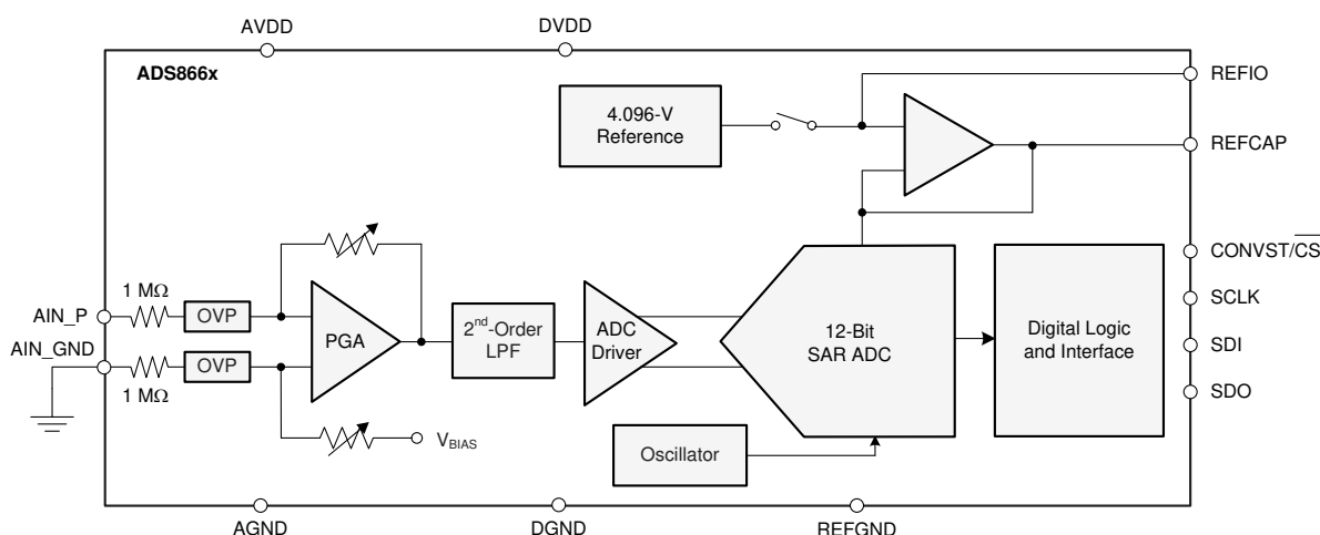
ブロック図
