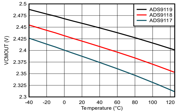
図 6-14. VCMOUT 電圧と温度との関係
