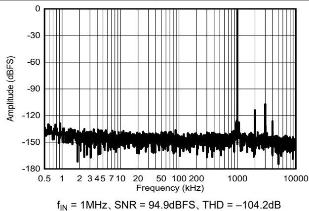
図 6-21. f_{IN} = 1\text{MHz} の標準 FFT
