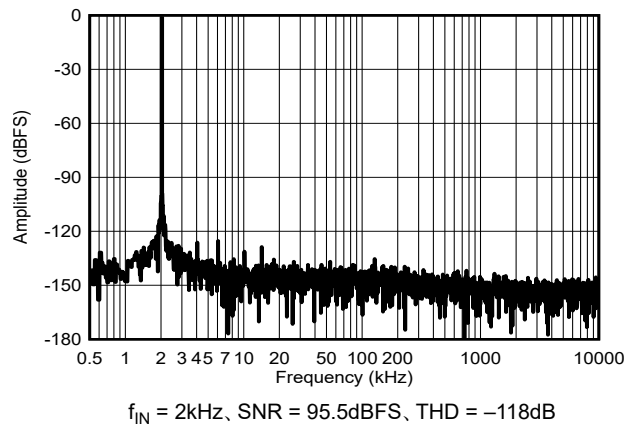
図 6-19. f_{IN} = 2\text{kHz} の標準 FFT
