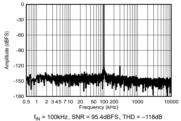
図 6-20. f_{IN} = 100\text{kHz} の標準 FFT
