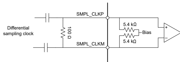
図 7-11. AC 結合差動サンプリング クロック
