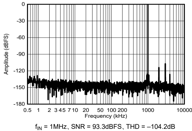
図 5-21. f_{IN} = 1\text{MHz} の標準 FFT
