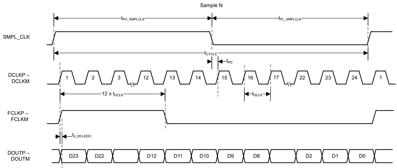
図 5-2. LVDS データ インターフェイス : SDR
