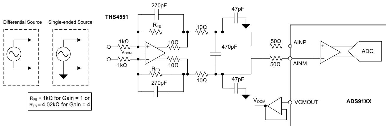
図 8-4. ≤100kHz の入力信号帯域幅のデータ アクイジション (DAQ) 回路
