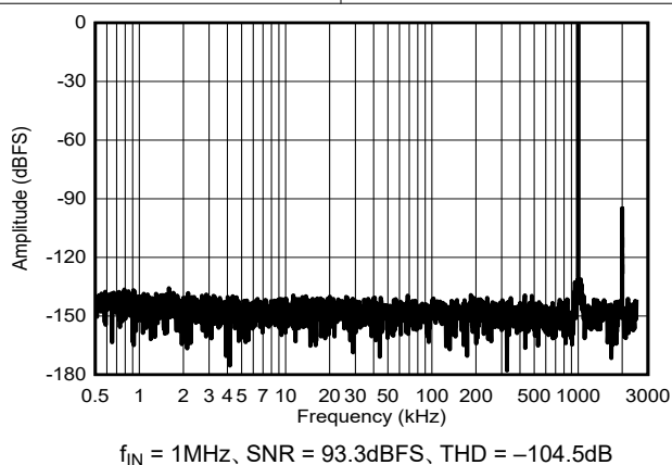
図 5-31. f_{IN} = 1\text{MHz} の標準 FFT
