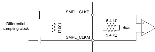
図 6-8. AC 結合差動サンプリングクロック
