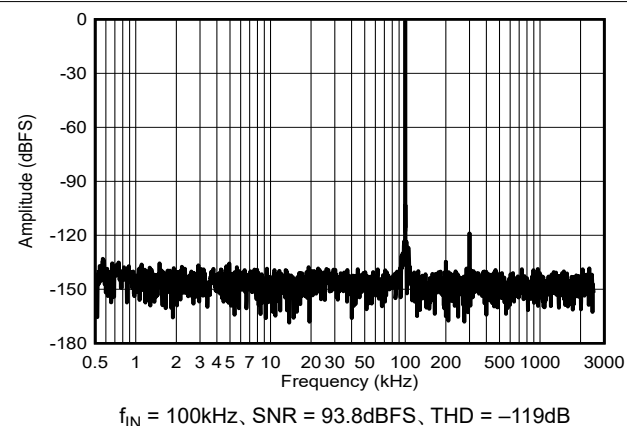
図 5-30. f_{IN} = 100\text{kHz} の標準 FFT
