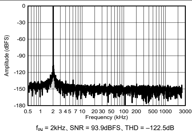
図 5-29. f_{IN} = 2\text{kHz} の標準 FFT
