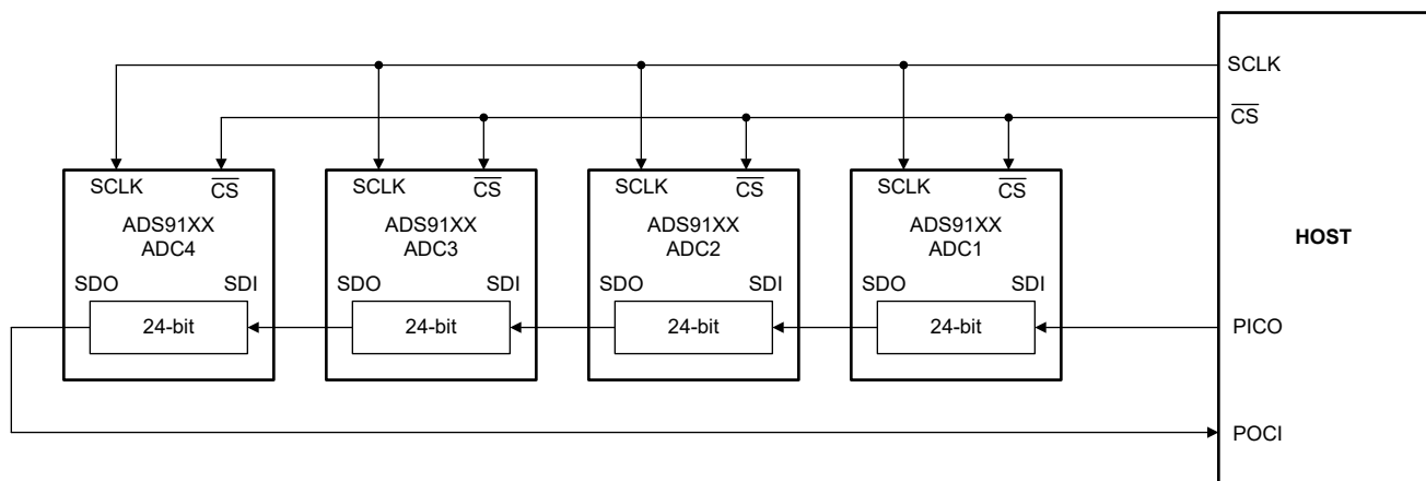
図 6-12. SPI 構成のデ이지チェーン接続
