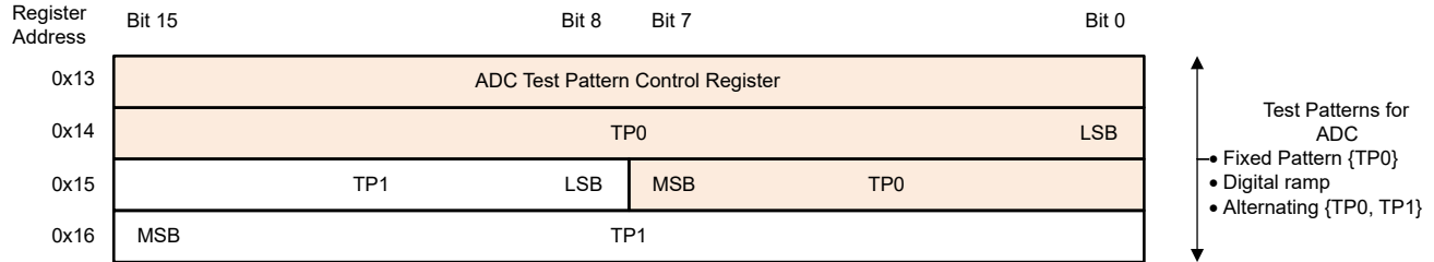
図 6-7. テスト パターンのレジスタ バンク
