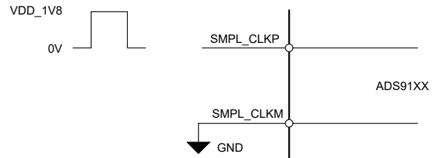
図 6-9. シングルエンド サンプリングクロック
