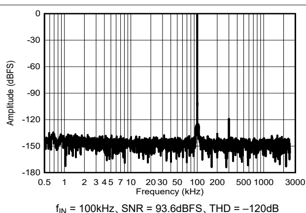
図 8-6. 5MSPS での標準 FFT: ADS9127
