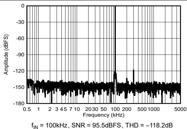
図 6-27. f_{IN} = 100\text{kHz} の標準 FFT
