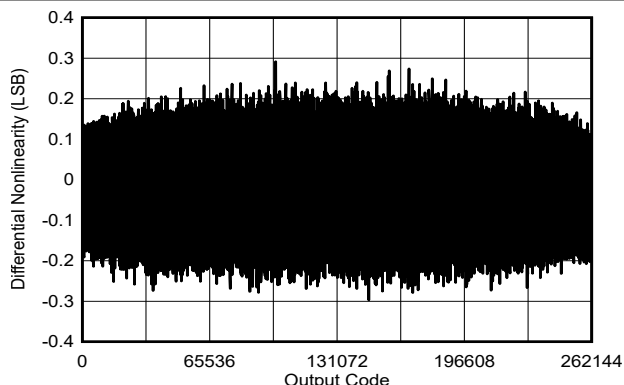
図 6-20. 標準 DNL
