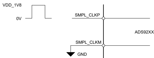
図 7-12. シングルエンド サンプルング クロック
