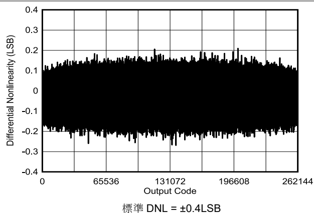
図 6-25. 標準 DNL
