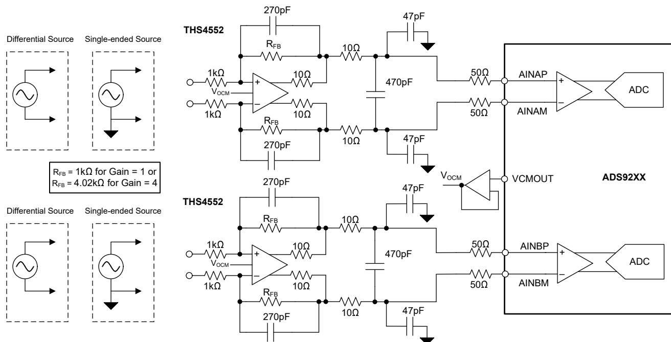
図 9-4. \leq 100\text{kHz} の入力信号帯域幅のデータ アクイジション (DAQ) 回路
