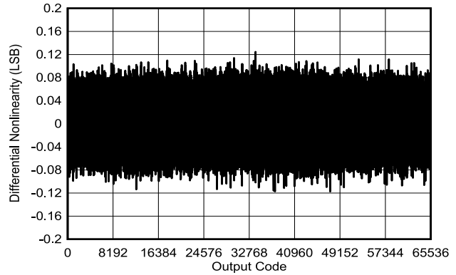
図 6-25. 標準 DNL
