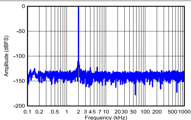
図 5-9. 広帯域幅 LPF を用いた標準的な FFT、 範囲 = \pm 5V
