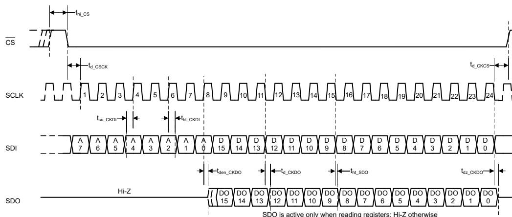
図 5-1. SPI 構成インターフェイス
