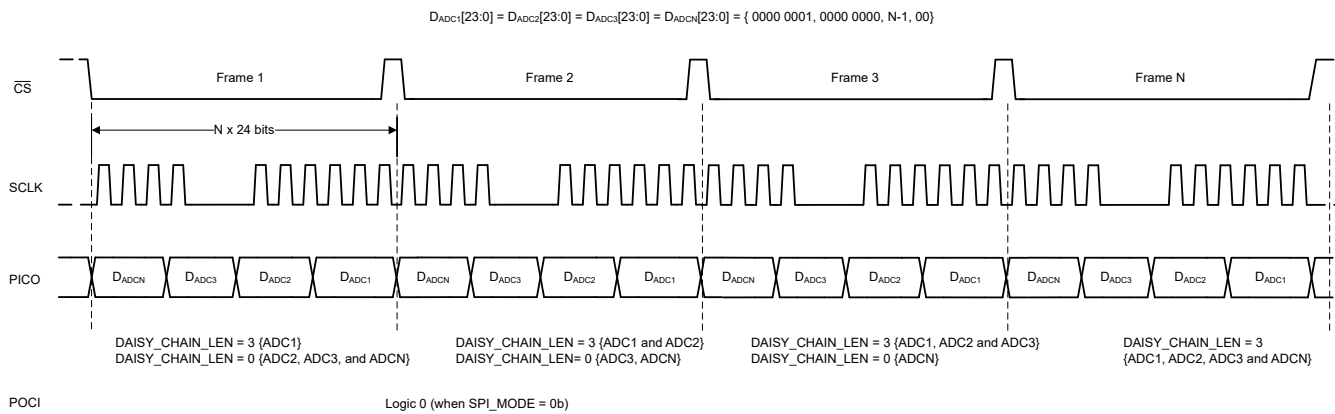
図 6-15. デイジーチェーンの長さを構成するためのレジスタ書き込み
