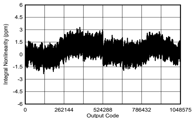
図 5-6. 標準 INL
