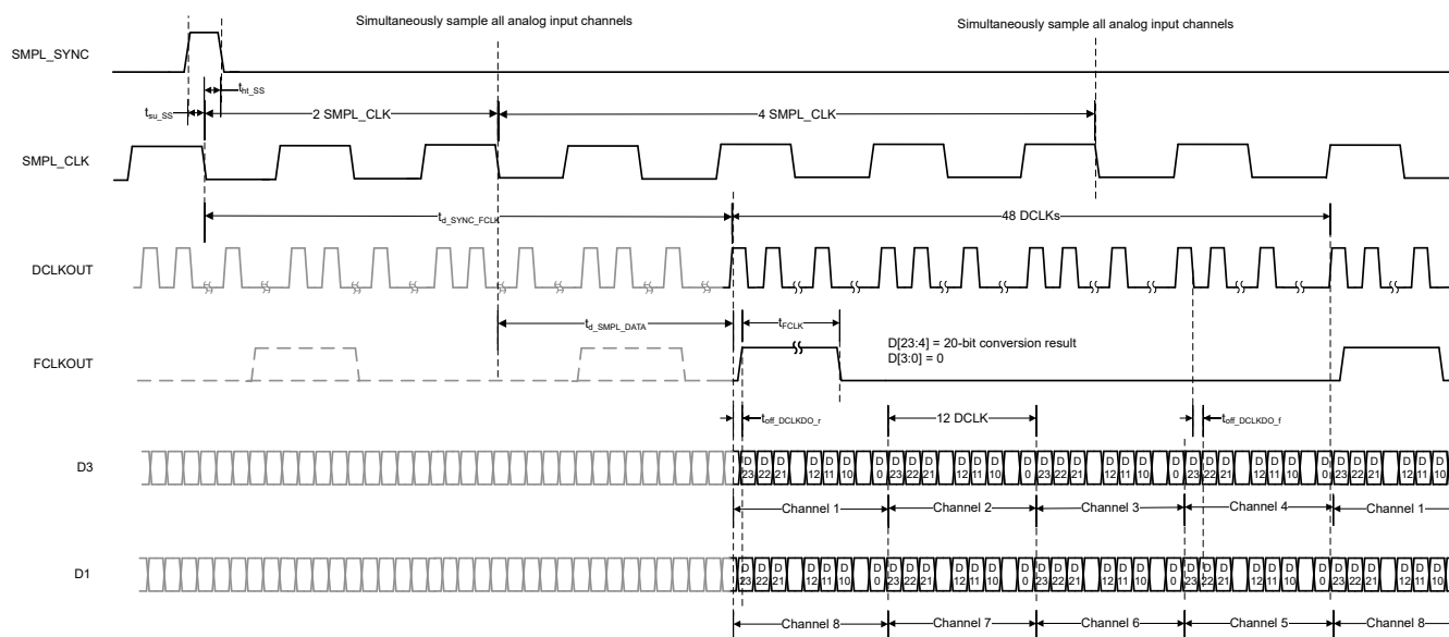
図 5-3. 2-SDO DDR CMOS データ インターフェイス
