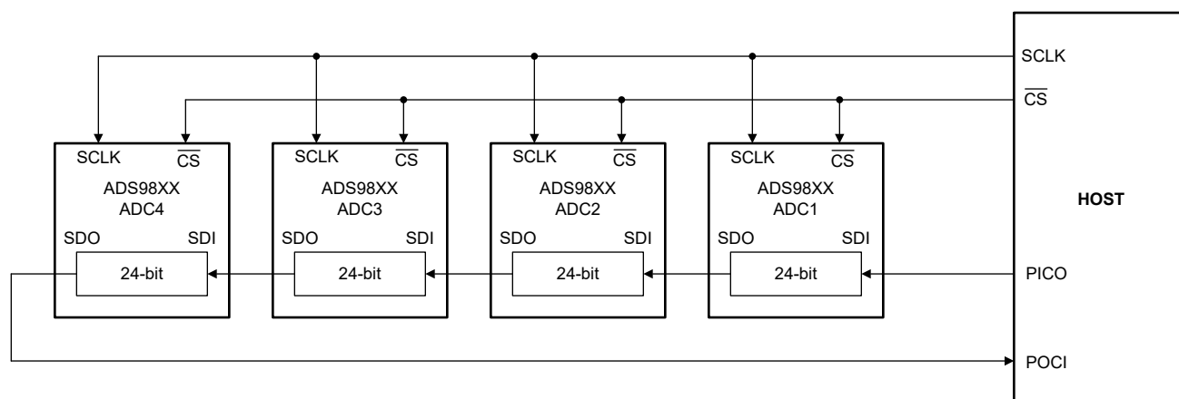
図 6-13. SPI 構成のデジタイズチェーン接続
