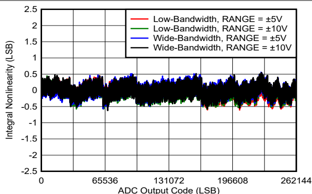
図 5-6. Typical INL
