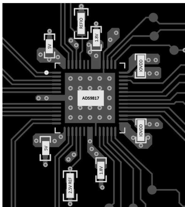
図 8-5. Example Layout
