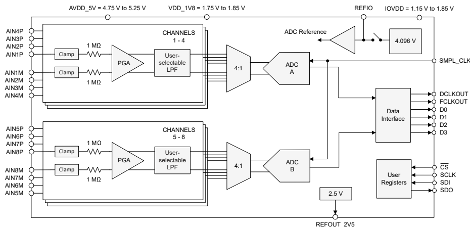
デバイスのブロック図
