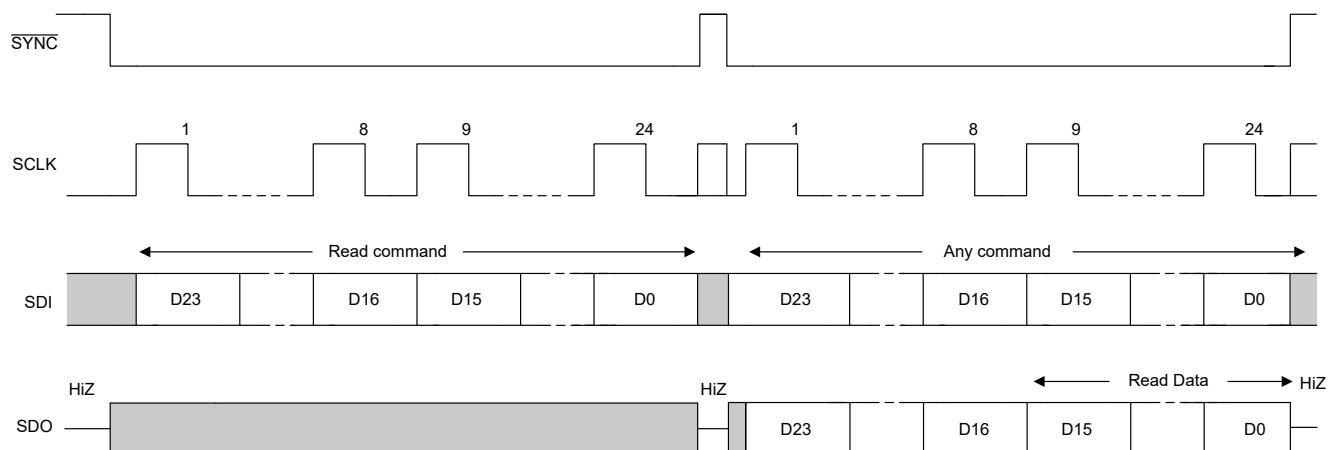
图 7-11. SPI Read Cycle
