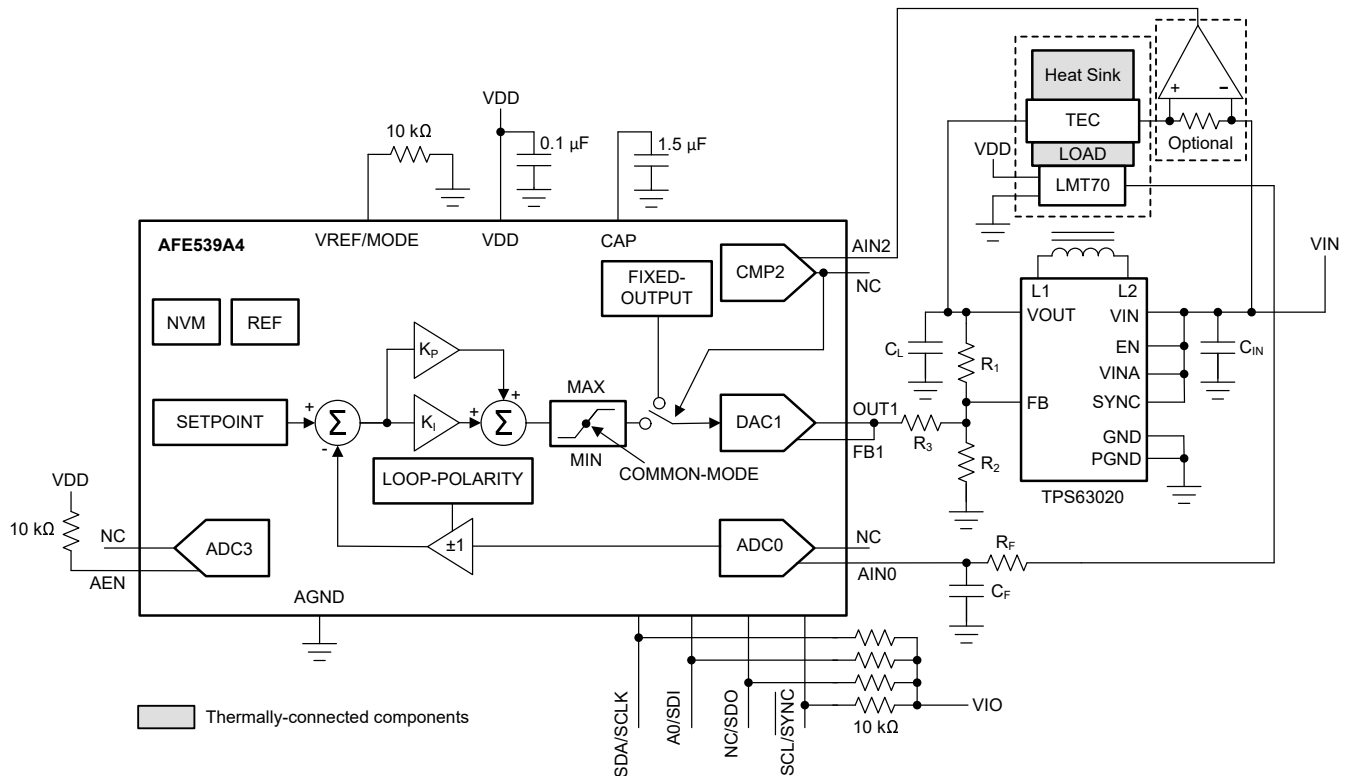
図 8-1. TEC Control
