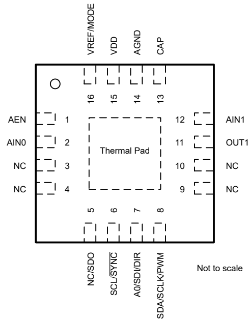
図 5-3. AFE439A2: RTE Package, 16-pin WQFN (Top View)
