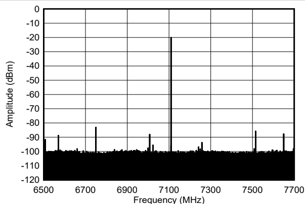
図 4-582. 7.1GHz、-12dBFS でのシングル トーン出カスペクトル (ナロー スパン)
