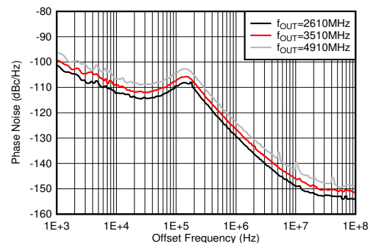
図 4-617. 9GHz VCO の位相ノイズとオフセット周波数との関係 (各種 f_{\text{OUT}} 、 25^\circ\text{C} )
