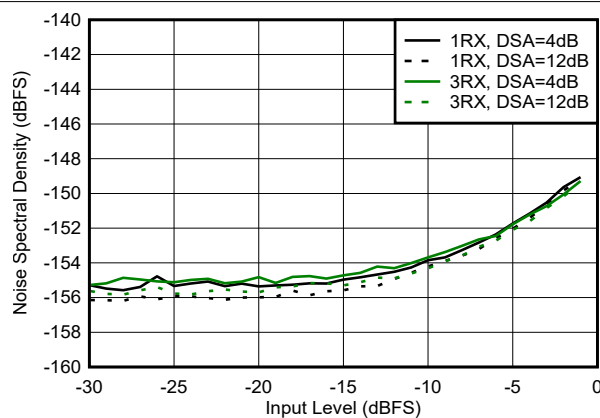
3.5GHz 整合あり、トーンから 12.5MHz オフセット
