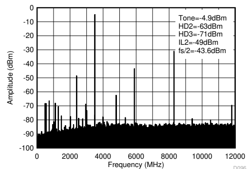
図 4-487. TX シングル トーン (-6dBFS) 出力スペクトル (3.5GHz, 0-f_{\text{DAC}} )
