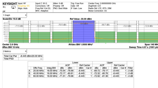
図 4-402. TX 20MHz LTE 出力スペクトル (バンド 41、2.6GHz)
