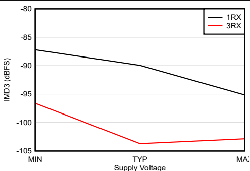
1.8GHz 整合あり、各トーン -7\text{dBFS} 、 20\text{MHz} のトーン間隔、すべての電源電圧は推奨動作条件の最小値、代表値、最大値
