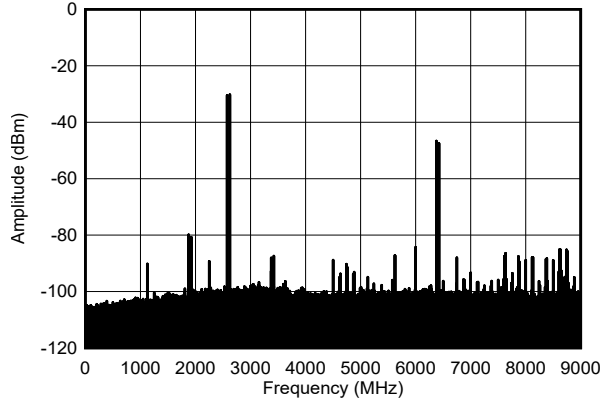
図 4-432. 2.6GHz での TX デュアル トーン出力スペクトル、各 -30dBFS (0 - f_{\text{DAC}} )
