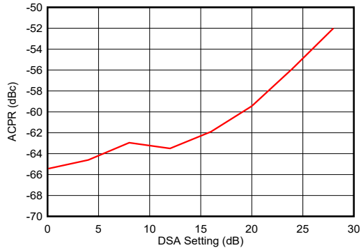
図 4-335. TX 100MHz NR ACPR と DSA との関係 (0.85GHz)
