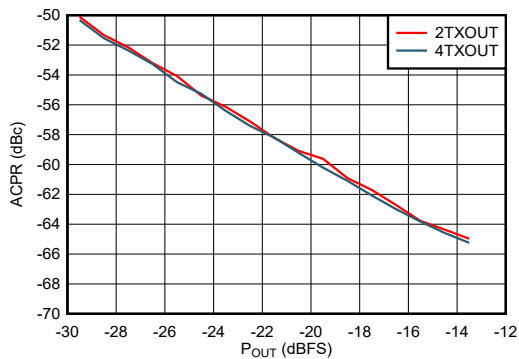
図 4-404. TX 20MHz LTE alt-ACPR とデジタル レベルとの関係 (2.6GHz)
