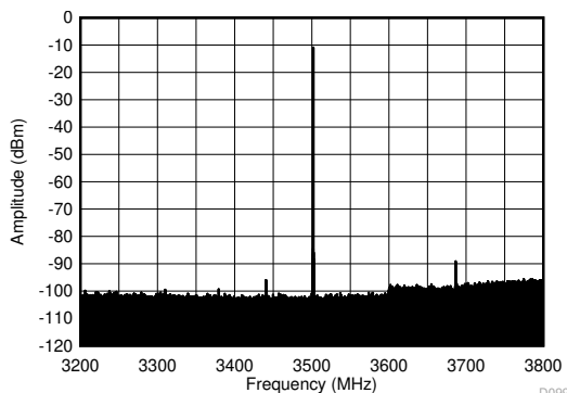
図 4-490. 3.5GHz での TX シングル トーン (-12dBFS) 出力スペクトル ( \pm 300\text{MHz} )
