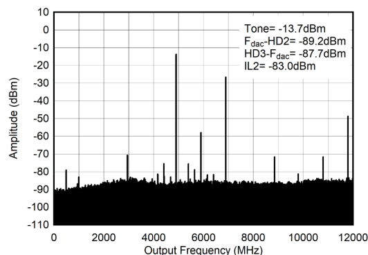
図 4-539. TX シングル トーン (-6dBFS) 出力スペクトル (4.9GHz、 0-f_{\text{DAC}} )
