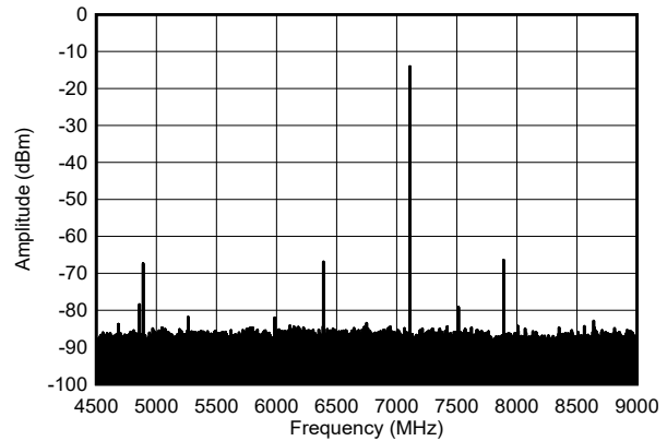
図 4-579. 7.1GHz、-6dBFS でのシングル トーン出カスペクトル (ナイキスト)
