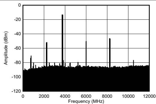
図 4-491. 3.75GHz での TX デュアル トーン出力スペクトル (各 -7dBFS、 0 \sim f_{\text{DAC}} )
