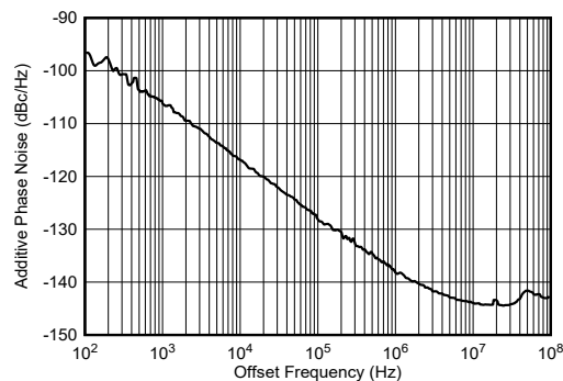
図 4-497. 3.7GHz での外部クロック付加位相ノイズ
