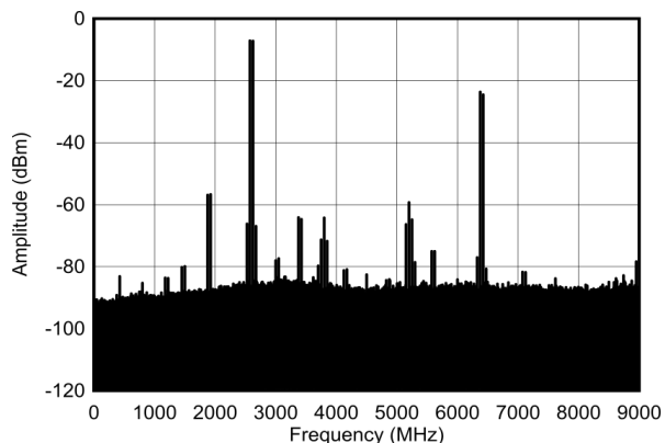
図 4-428. 2.6GHz での TX デュアル トーン出力スペクトル、各 -7dBFS (0 - DAC)
