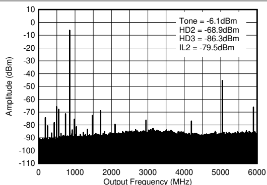
図 4-345. TX シングル トーン (-1dBFS) 出力スペクトル (0.85GHz、 0-f_{\text{DAC}} )
