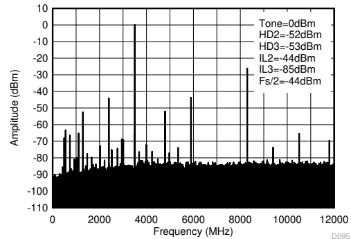
図 4-485. TX シングル トーン (-1dBFS) 出力スペクトル (3.5GHz, 0-f_{\text{DAC}} )
