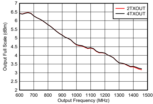
図 4-293. TX フルスケールと RF 周波数の関係 (各種チャネル、5898.24MSPS、ストレート モード)
