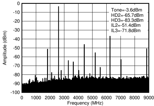
図 4-416. TX シングル トーン (-12dBFS) 出力スペクトル (2.6GHz, 0-f_{\text{DAC}} )
