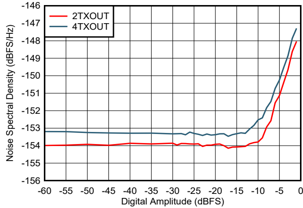
図 4-574. 7.1GHz での NSD とデジタル振幅とチャンネルとの関係
