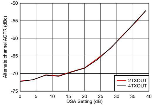
図 4-359. TX 20MHz LTE alt-ACPR と DSA との関係 (1.8GHz)
