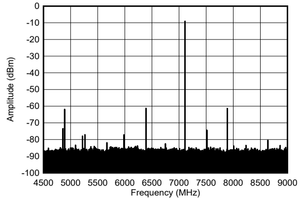
図 4-577. 7.1GHz、-1dBFS でのシングル トーン出力スペクトル (ナイキスト)
