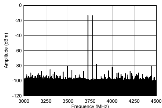
図 4-492. 3.75GHz での TX デュアル トーン出力スペクトル、各 -7dBFS ( \pm 600\text{MHz} )
