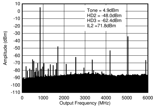
図 4-349. TX シングル トーン (-6dBFS) 出力スペクトル (0.85GHz、 0-f_{\text{DAC}} )
