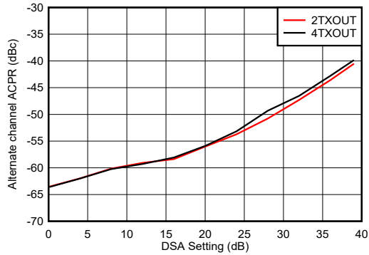
図 4-534. TX 100MHz NR alt-ACPR と DSA との関係 (4.9GHz)
