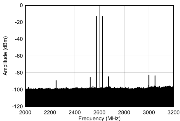
図 4-429. 2.6GHz での TX デュアル トーン出力スペクトル、各 -7dBFS (±600MHz)
