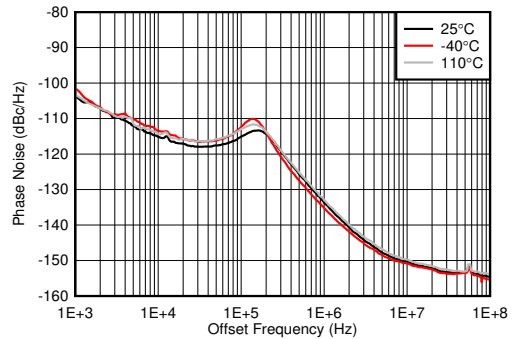
図 4-603. 12GHz VCO の位相ノイズと温度との関係 (各種 f_{\text{REF}} 、 f_{\text{OUT}} = 2.6\text{GHz} 、5MHz オフセット)
