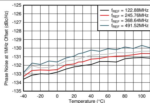
図 4-601. 12GHz VCO の位相ノイズと温度との関係 (各種 f_{\text{REF}} 、 f_{\text{OUT}} = 2.6\text{GHz} 、 1\text{MHz} オフセット)
