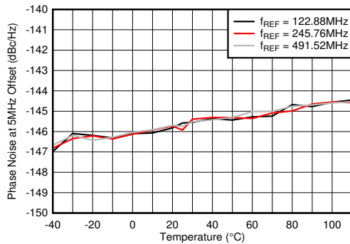
図 4-614. 10GHz VCO の位相ノイズと温度との関係 (各種 f_{\text{REF}} 、 f_{\text{OUT}} = 2.6\text{GHz} 、5MHz オフセット)
