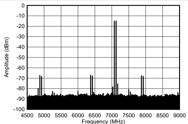
図 4-581. 7.1GHz、-12dBFS でのシングル トーン出カスペクトル (ナイキスト)
