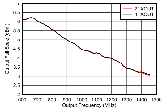
図 4-294. TX フルスケールと RF 周波数の関係 (各種チャネル、8847.36MSPS、ストレート モード)
