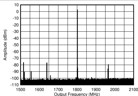
図 4-372. TX シングル トーン (-1dBFS) 出力スペクトル (1.8GHz、0- f_{\text{DAC}} )
