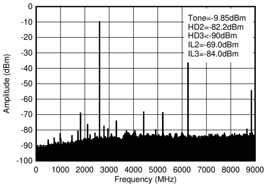
図 4-420. TX シングル トーン (-1dBFS) 出力スペクトル (2.6GHz, 0- f_{\text{DAC}} )
