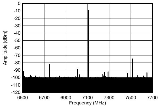
図 4-578. 7.1GHz、-1dBFS でのシングル トーン出カスペクトル (ナロー スパン)
