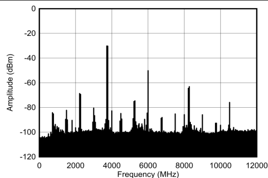
図 4-493. 3.75GHz での TX デュアル トーン出力スペクトル (各 -13dBFS、 0 \sim f_{\text{DAC}} )
