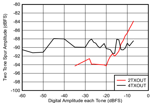
帯域内 = 2600\text{MHz} \pm 600\text{MHz} 、 f_{DAC} = 12\text{GSPS} 、 F_S/3 および F_S/4 を含まず、外部クロック モード、非インターリーブ モード
