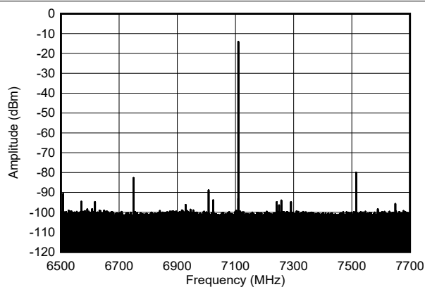
図 4-580. 7.1GHz、-6dBFS でのシングル トーン出カスペクトル (ナロー スパン)
