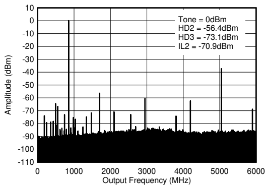
図 4-341. TX シングル トーン (-12dBFS) 出力スペクトル (0.85GHz、0- f_{\text{DAC}} )
