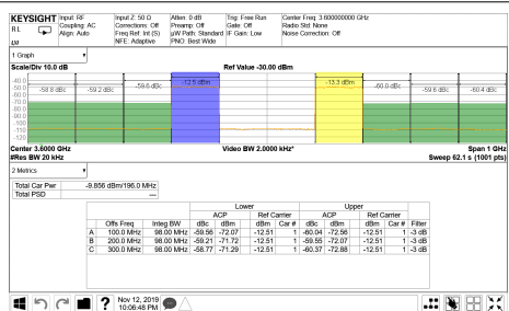
3.5GHz 整合あり、シングル キャリア 100MHz BW NR TM1.1
