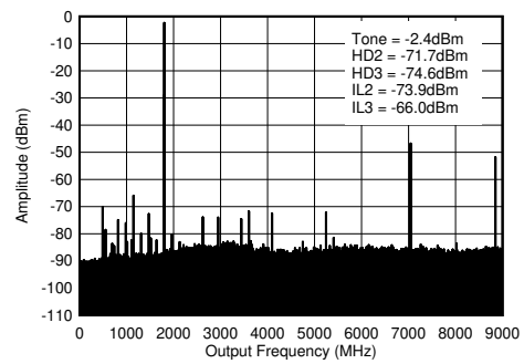
図 4-368. TX シングル トーン (-12dBFS) 出力スペクトル (1.8GHz、 0-f_{\text{DAC}} )
