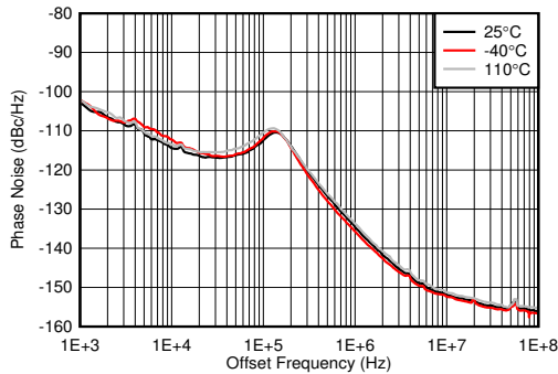
図 4-614. 10GHz VCO の位相ノイズと温度との関係 (各種 f_{\text{REF}} 、 f_{\text{OUT}} = 2.6\text{GHz} 、5MHz オフセット)
