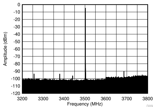
図 4-486. 3.5GHz での TX シングル トーン (-1dBFS) 出力スペクトル ( \pm 300\text{MHz} )
