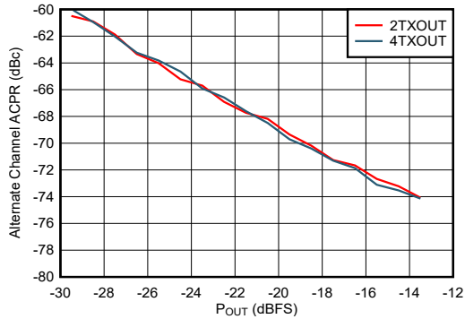
図 4-404. TX 20MHz LTE alt-ACPR とデジタル レベルとの関係 (2.6GHz)
