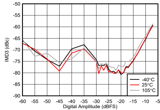
図 4-439. 2.6GHz での IMD3 とデジタル振幅と温度との関係
