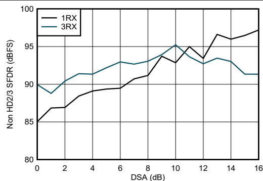
図 4-77. RX (HD2/3 を除く) と DSA 設定との関係 (0.8GHz)
