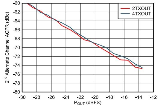
図 4-405. TX 20MHz LTE alt2-ACPR とデジタル レベルとの関係 (2.6GHz)
