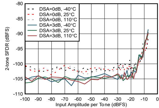
図 4-168. RX 2 トーン SFDR と入力振幅、DSA 設定との関係 (3.7GHz)
