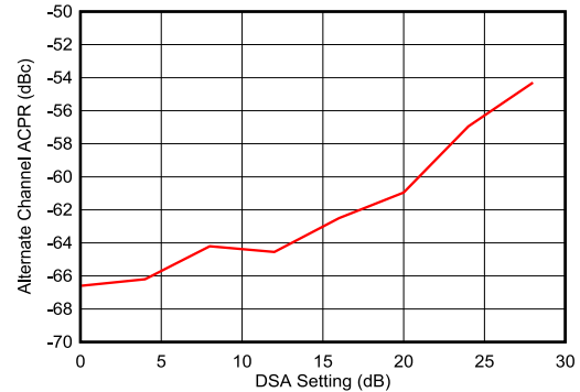
図 4-336. TX 100MHz NR alt-ACPR と DSA との関係 (0.85GHz)
