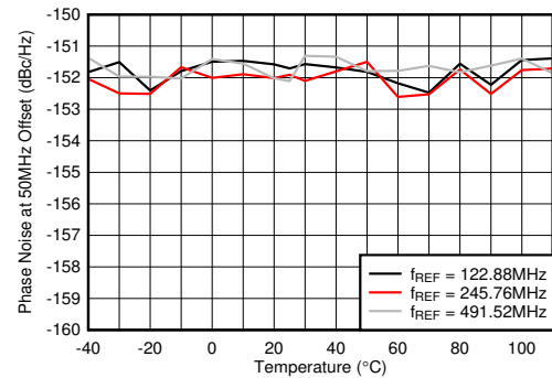
図 4-615. 10GHz VCO の位相ノイズと温度との関係 (各種 f_{\text{REF}} 、 f_{\text{OUT}} = 2.6\text{GHz} 、50MHz オフセット)
