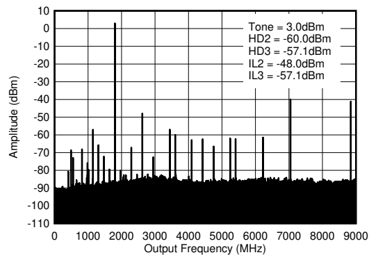
図 4-364. TX シングル トーン (-6dBFS) 出力スペクトル (1.8GHz、 0-f_{\text{DAC}} )
