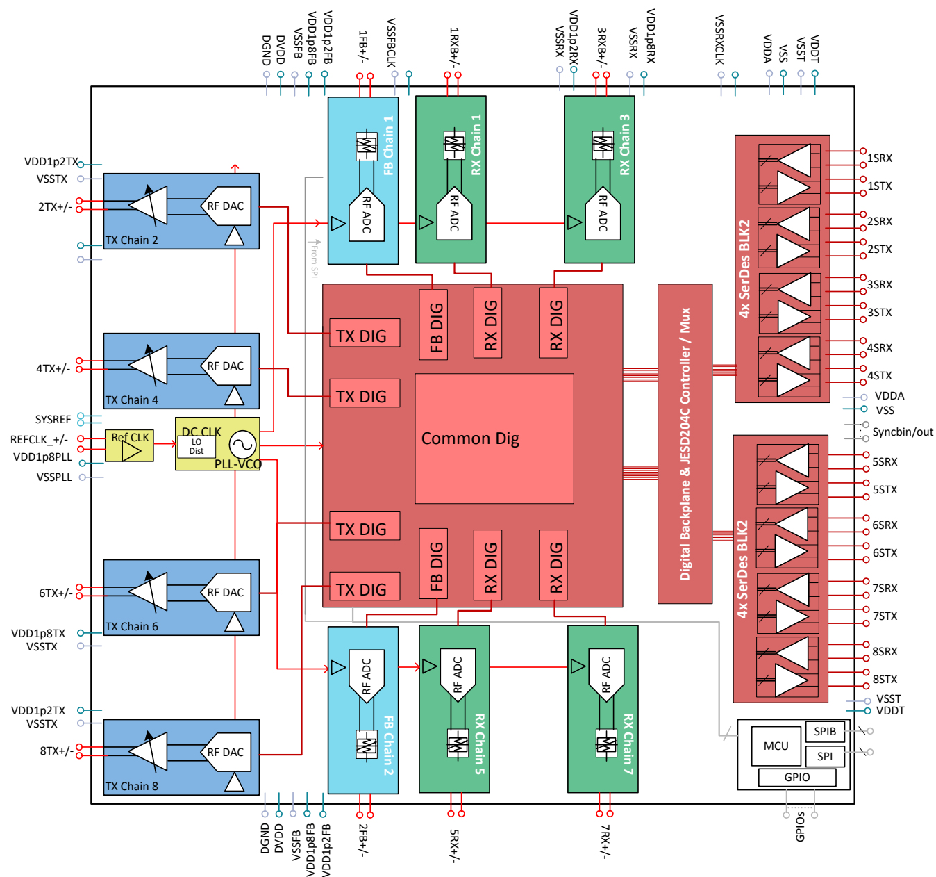
AFE8124 の機能ブロック図
