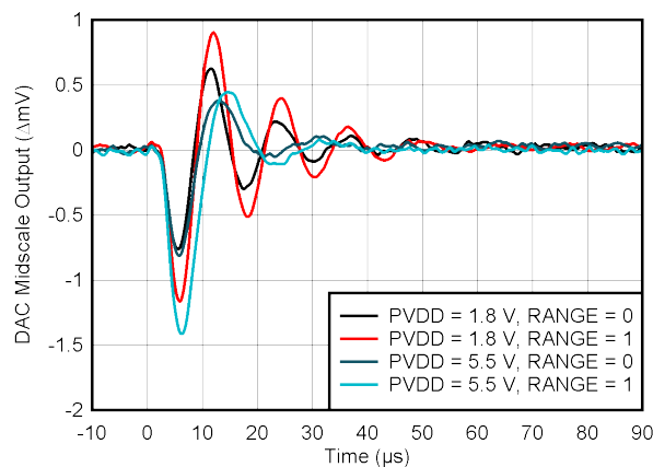
FIG 6-25. DAC Glitch Impulse Rising Edge
