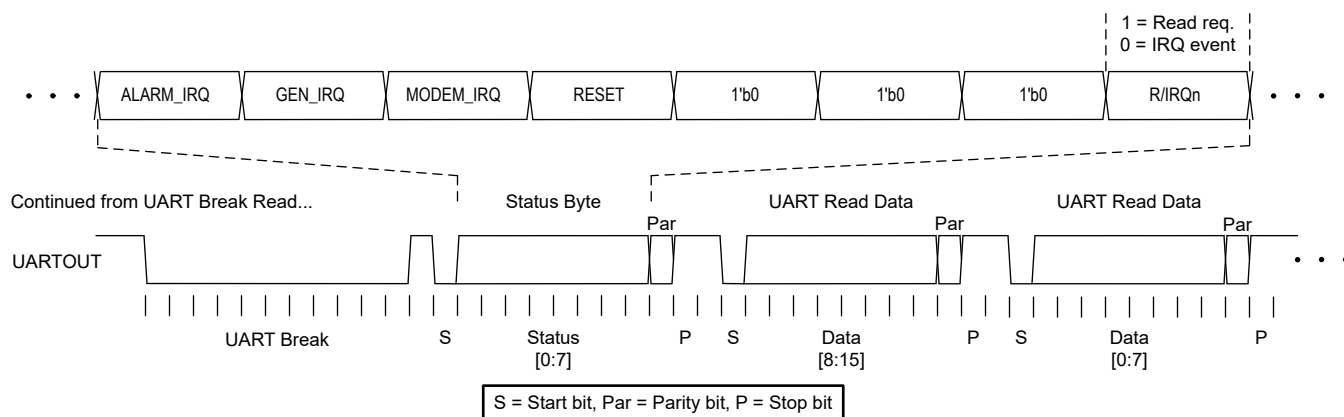
7-33. UARTOUT Break Data Format
