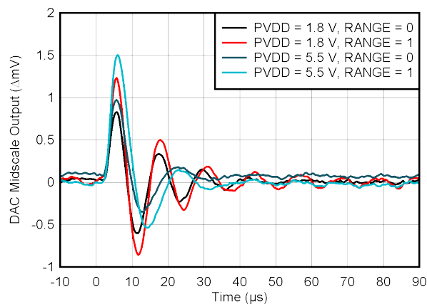
FIG 6-26. DAC Glitch Impulse Falling Edge
