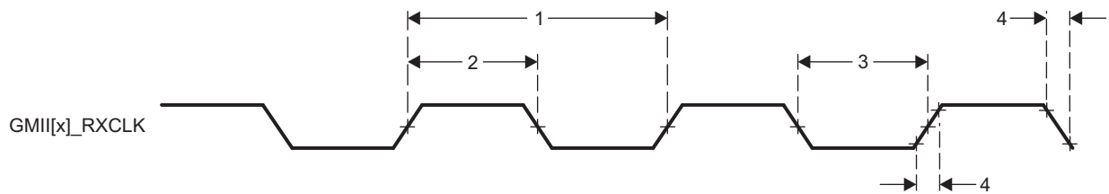
図 7-6. GMII[x]_RXCLK Timing - MII Mode
