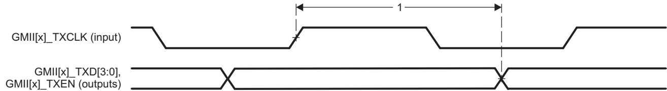
図 7-9. GMII[x]_TXD[3:0], GMII[x]_TXEN Timing - MII Mode
