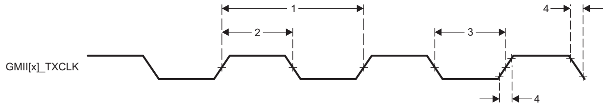
図 5-23. GMII[x]_TXCLK Timing - MII Mode
