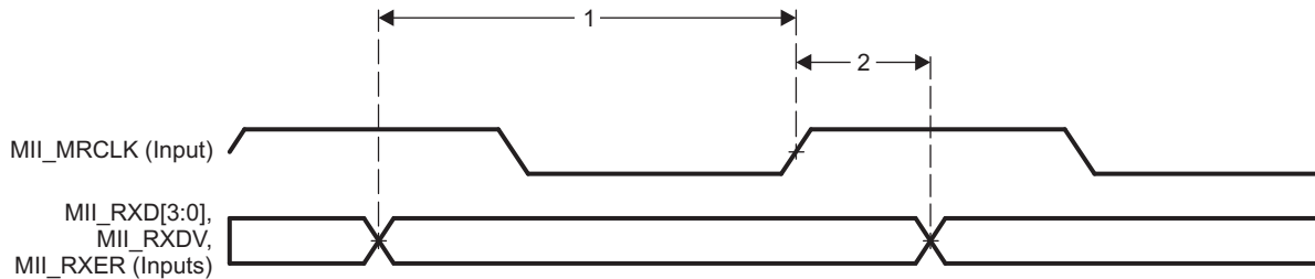
図 5-137. PRU-ICSS MII_RXD[3:0], MII_RXDV, and MII_RXER Timing
