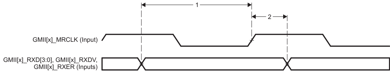
図 5-24. GMII[x]_RXD[3:0], GMII[x]_RXDV, GMII[x]_RXER Timing - MII Mode
