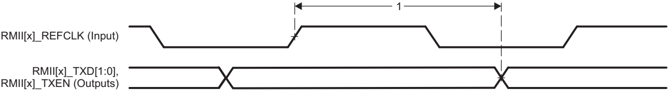
図 5-28. RMII[x]_TXD[1:0], RMII[x]_TXEN Timing - RMII Mode
