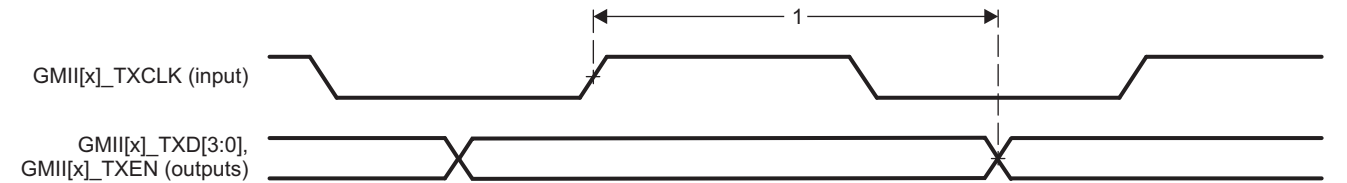
图 5-25. GMII[x]_TXD[3:0], GMII[x]_TXEN Timing - MII Mode
