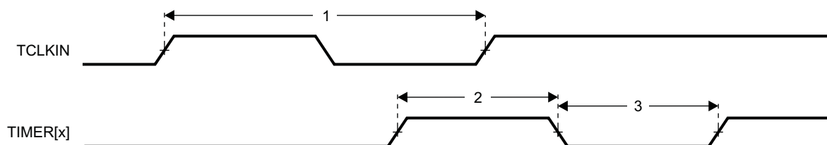
图 5-18. Timer Timing
