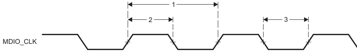
图 5-133. PRU-ICSS MDIO_CLK Timing
