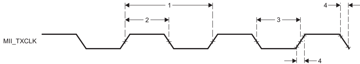
図 5-136. PRU-ICSS MII_TXCLK Timing
