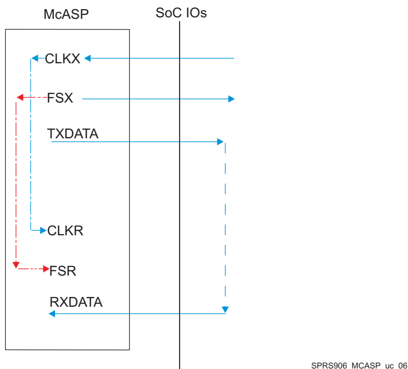
图 5-61. McASP1-8 CI-FO- – SYNC Mode
