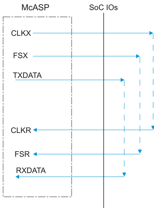
图 5-56. McASP1-8 COIFOI – ASYNC Mode
