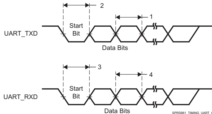
图 5-124. PRU-ICSS UART Timing
