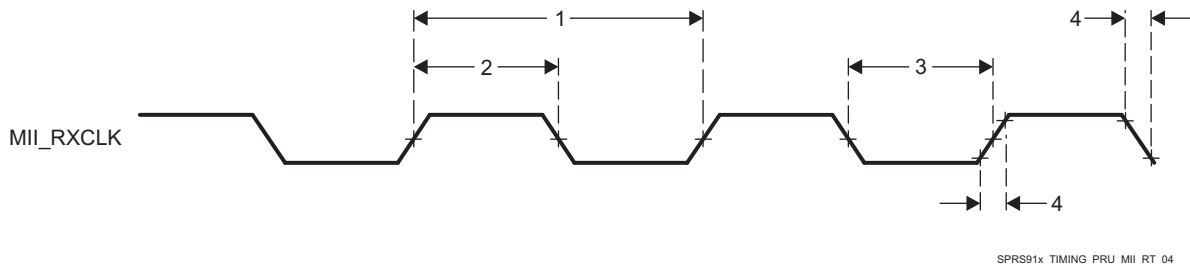
图 5-120. PRU-ICSS MII[x]_RXCLK Timing
