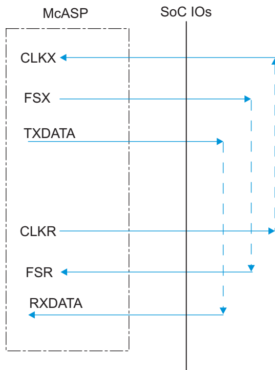
FIG 5-59. McASP1-8 CIOFOI – ASYNC Mode
