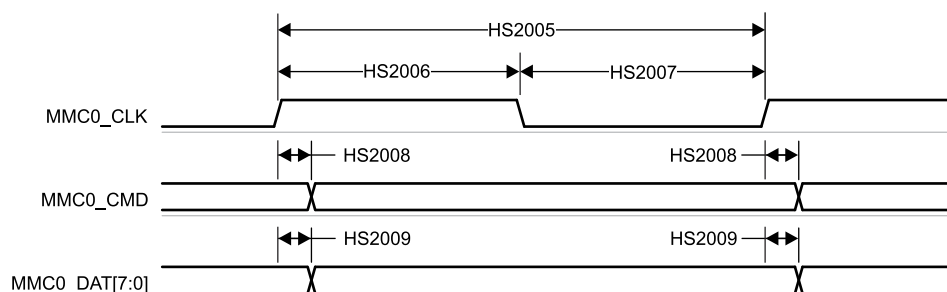
図 6-65. MMC0 – HS200 モード – 送信モード
