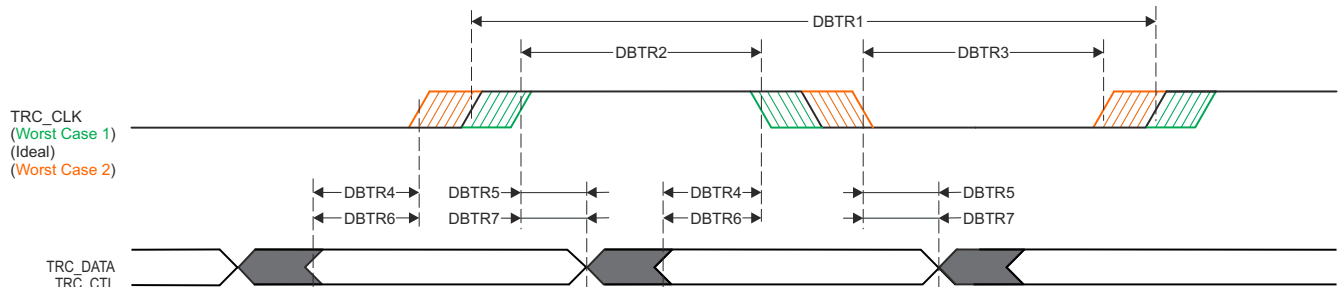
図 6-115. トレースのスイッチング特性
