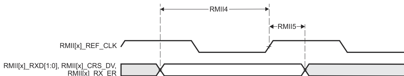
図 6-24. CPSW3G RMII[x]_RXD[1:0], RMII[x]_CRS_DV, RMII[x]_RX_ER のタイミング要件 - RMII モード
