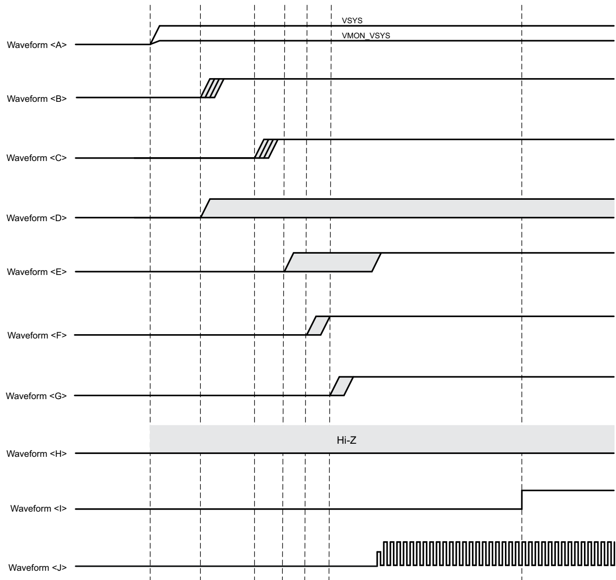
図 6-5. パワーアップ シーケンス
