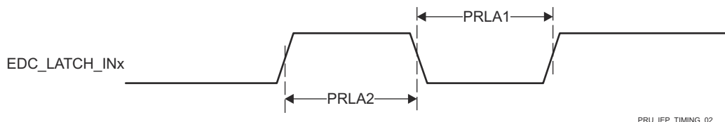
図 6-102. PRU_ICSSG IEP LATCH_INx のタイミング要件
