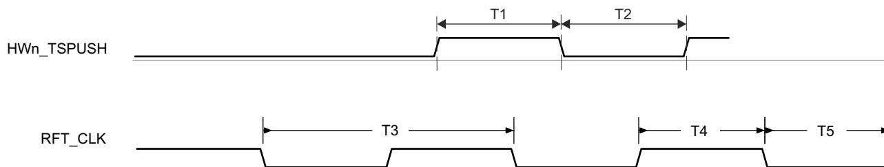
図 6-77. CPTS のタイミング要件
