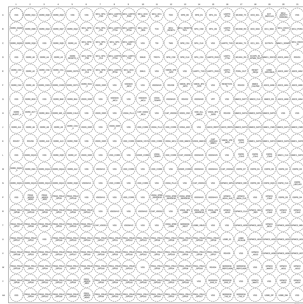
図 5-1. ALV/ANI FCBGA-N441 ピン配置図 (上面図)
