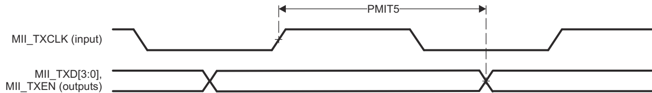
図 6-121. PRU_ICSSG MII_TXD[3:0], MII_TXEN Timing
