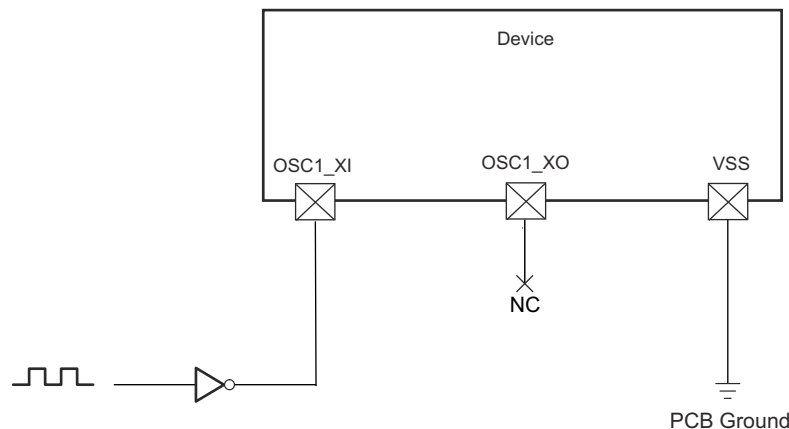
図 6-22. 1.8-V LVC MOS-Compatible Clock Input
