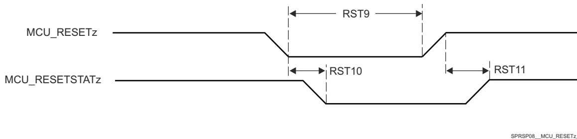
図 6-8. MCU_RESETz and MCU_RESETSTATz Timing
