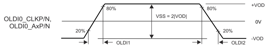
図 6-92. OLDI Data Output Jitter
