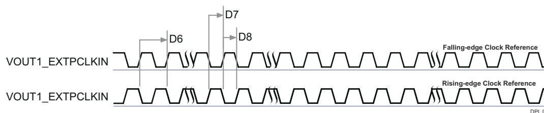
図 6-40. DPI External Pixel Clock Input
