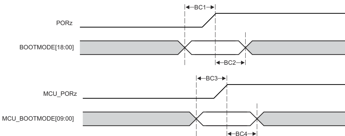
図 6-9. Boot Configuration Timing
