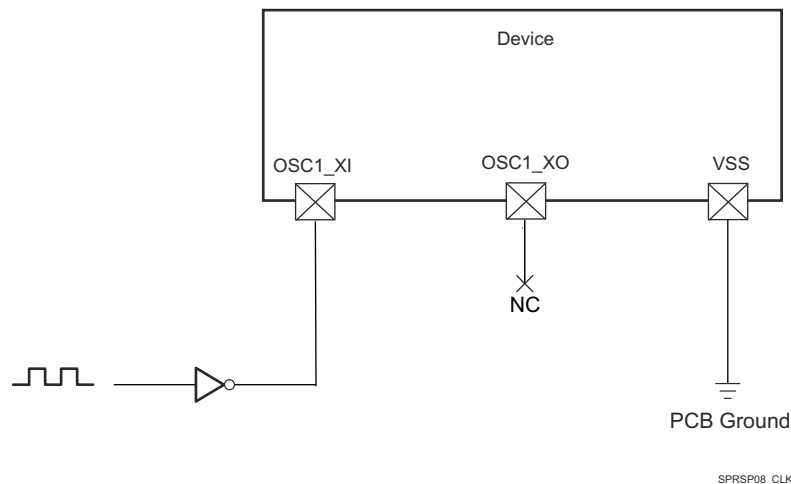
図 6-22. 1.8-V LVC MOS-Compatible Clock Input
