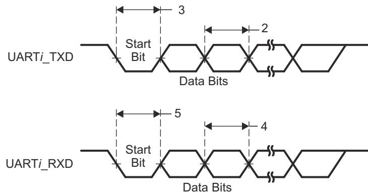
図 6-123. UART Timing
