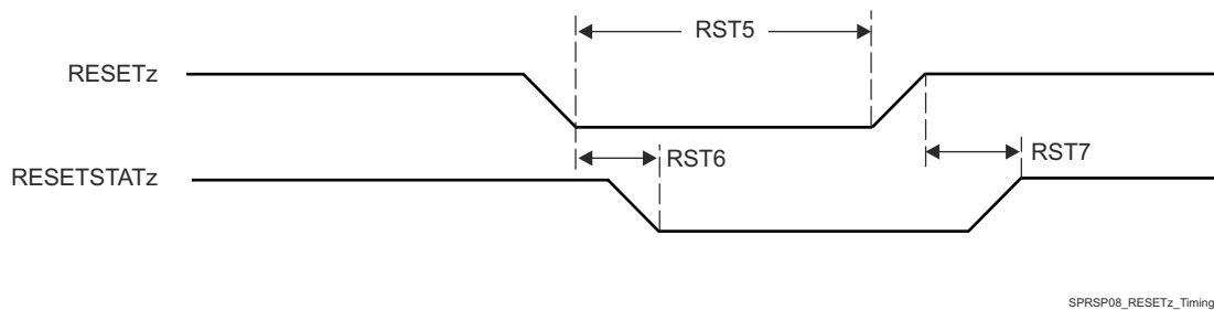
図 6-7. RESETz and RESETSTATz Timing
