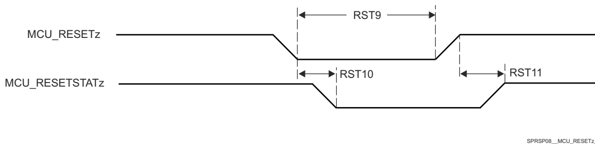
図 6-8. MCU_RESETz and MCU_RESETSTATz Timing
