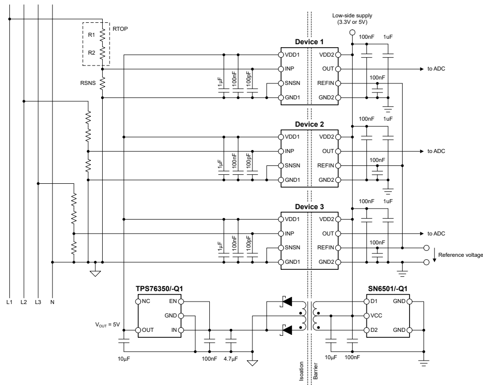
図 8-1. 代表的なアプリケーションで AMC0x30S を使用
