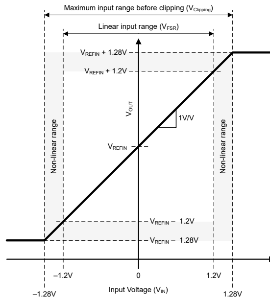
図 7-2. AMC0x30S の入力から出力への伝達曲線
