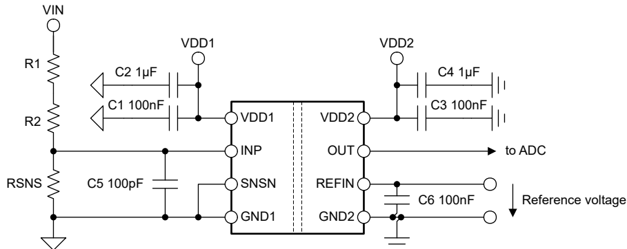
図 8-5. AMC0x30S のデカップリング
