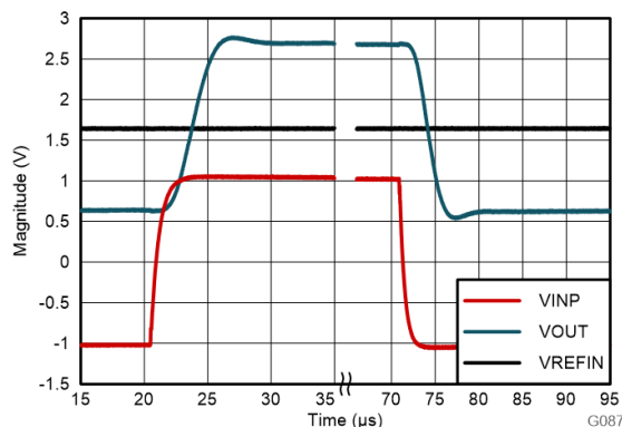
図 8-4. AMC0x30S のステップ応答
