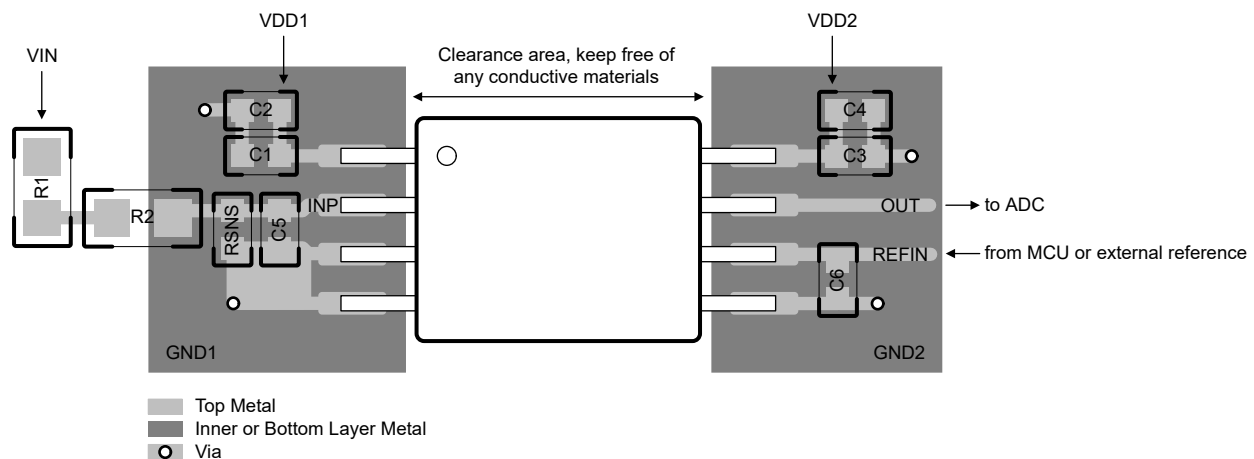
図 8-6. AMC0x30S の推奨レイアウト
