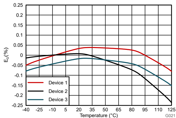
図 6-19. ゲイン誤差と温度との関係
