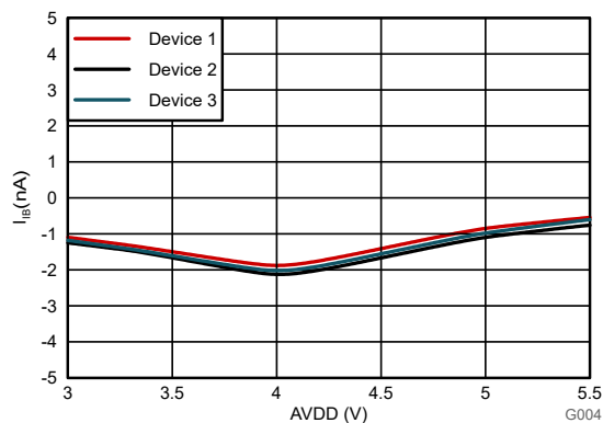
図 6-7. 入力バイアス電流とハイサイド電源電圧との関係 (INP ピン)
