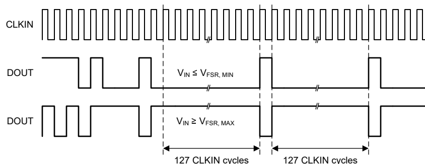
図 7-5. AMC0x36 のフルスケール出力
