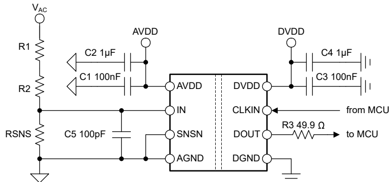
図 8-4. AMC0x36 のデカップリング
