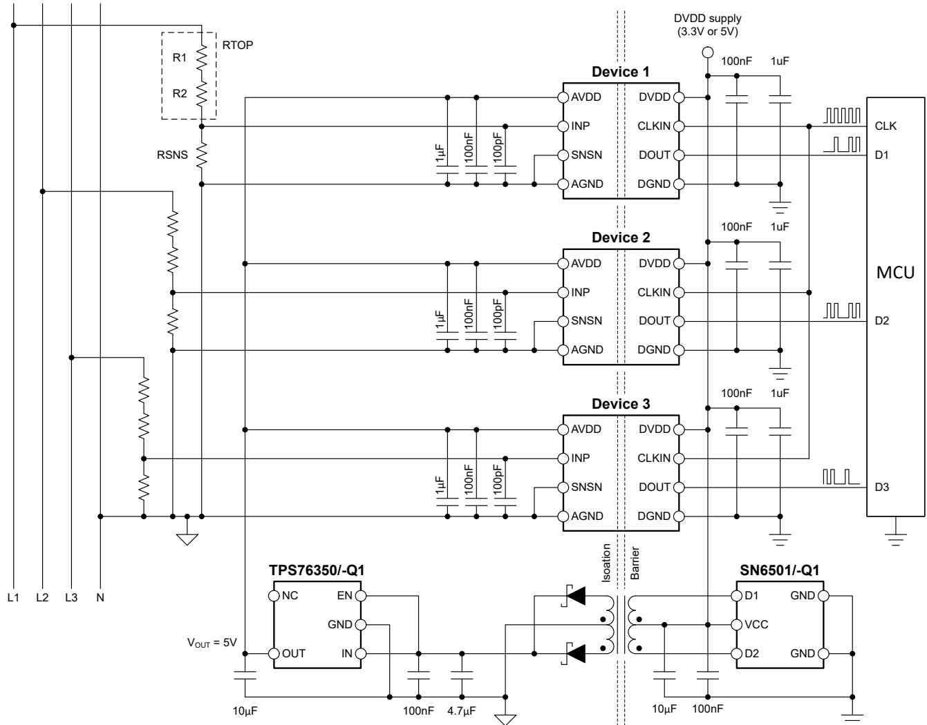
図 8-1. 代表的なアプリケーションで使用 AMC0x36
