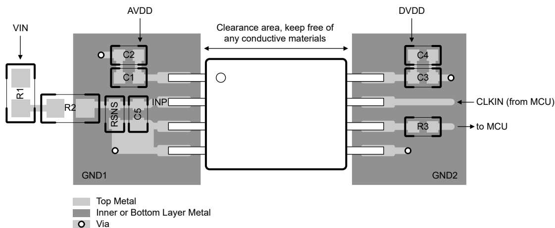
図 8-5. AMC0x36 の推奨レイアウト
