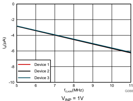
図 6-11. 入力バイアス電流とクロック周波数との関係 (SNSN ピン)
