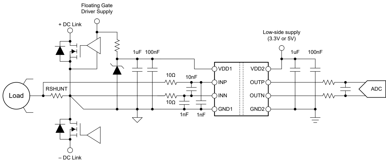
図 8-1. 代表的なアプリケーションでの電流検出に AMC0x00D を使用
