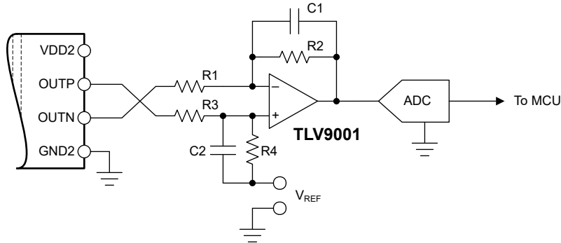
図 8-3. AMC0x00D 出力をシングルエンド入力 ADC に接続する
