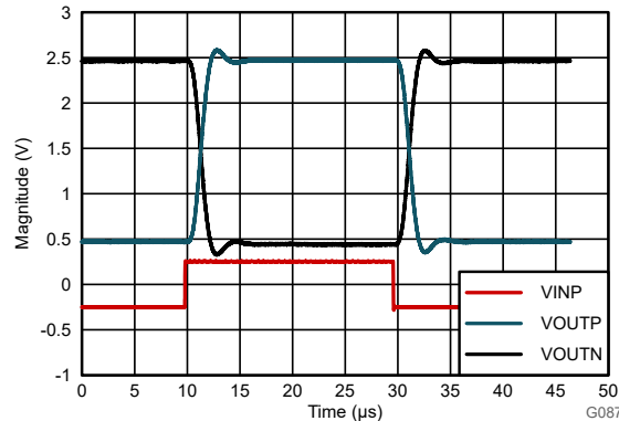
図 8-4. AMC0x00D のステップ応答
