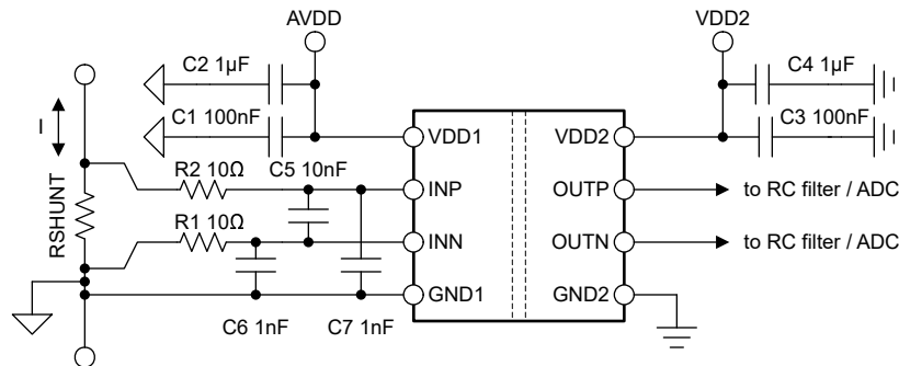
図 8-5. AMC0x00D のデカップリング
