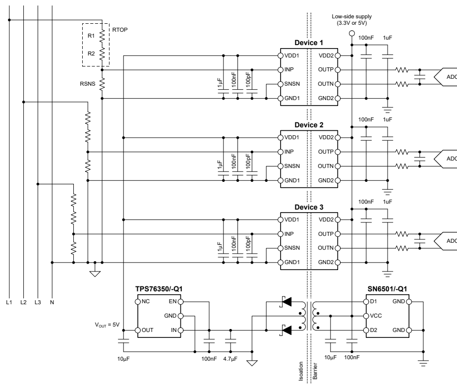
図 8-1. 代表的なアプリケーションで使用 AMC0x30D
