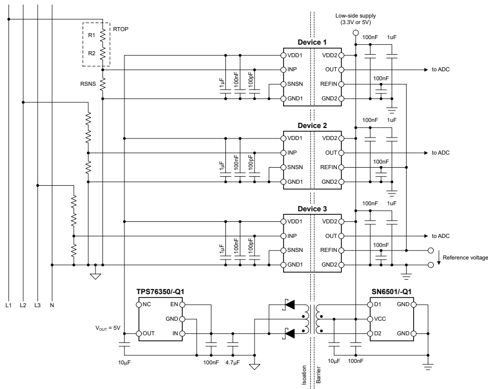
図 8-1. 代表的なアプリケーションで使用 AMC0x30R-Q1
