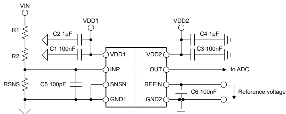
図 8-5. AMC0x30R-Q1 のデカップリング
