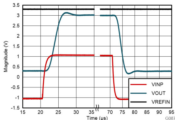
図 8-4. AMC0x30R-Q1 のステップ応答
