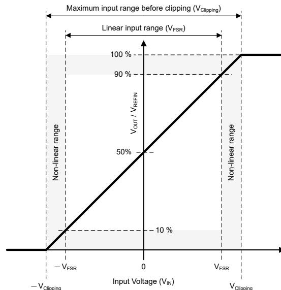
図 7-2. AMC0x30R-Q1 の入力から出力への伝達曲線
