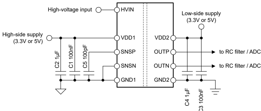
図 8-5. AMC0380D-Q1 のデカップリング
