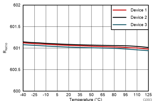
AMC0380D06-Q1
