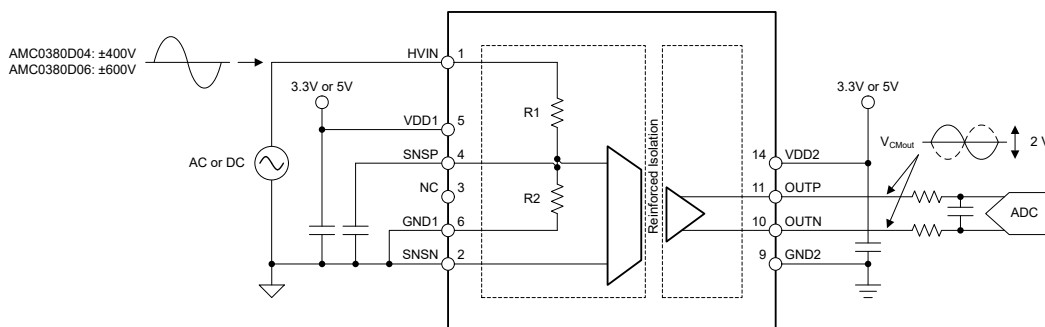
代表的なアプリケーション回路図 (DFX パッケージ)
