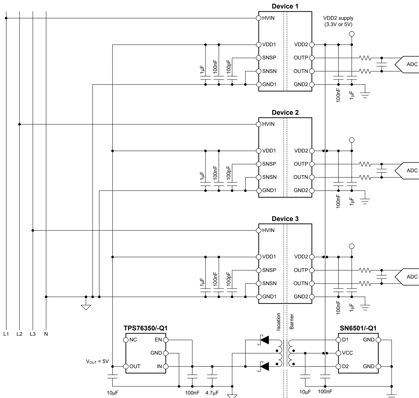
図 8-1. 代表的なアプリケーションで AMC0380D-Q1 を使用
