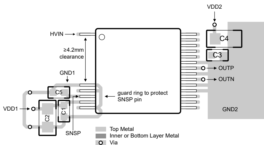
図 8-7. AMC0380D-Q1(DFJ パッケージ) の推奨レイアウト
