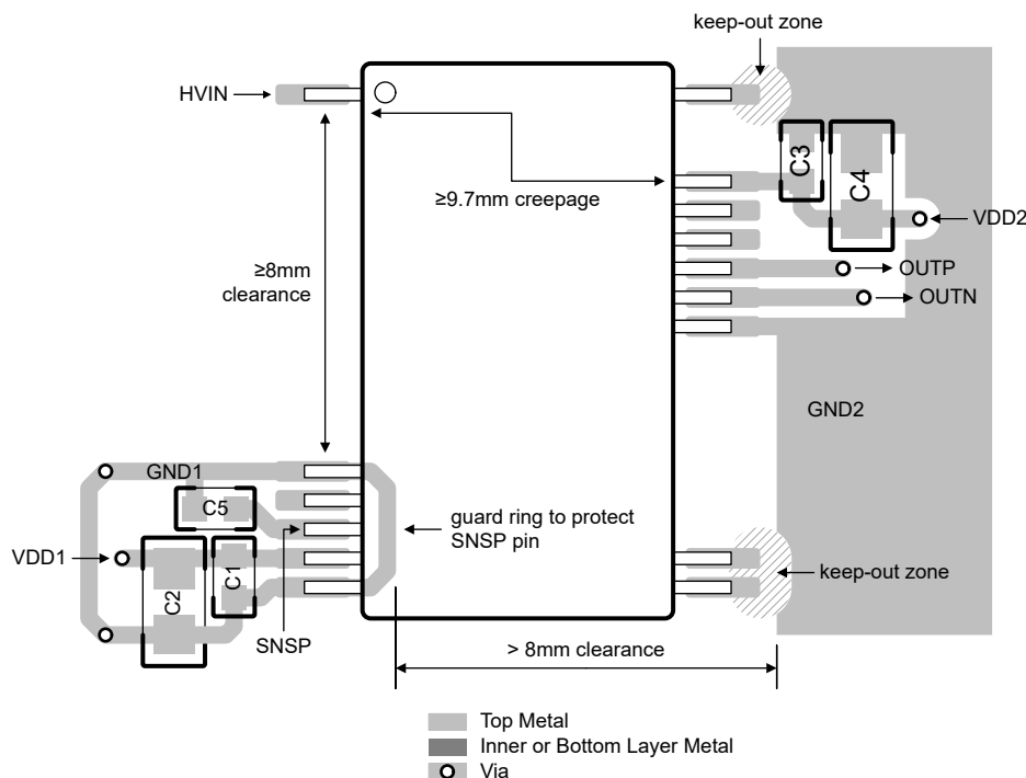
図 8-6. AMC0380D-Q1(DFX パッケージ) の推奨レイアウト
