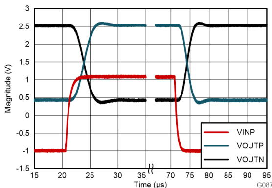
図 8-4. AMC0380D-Q1 のステップ応答
