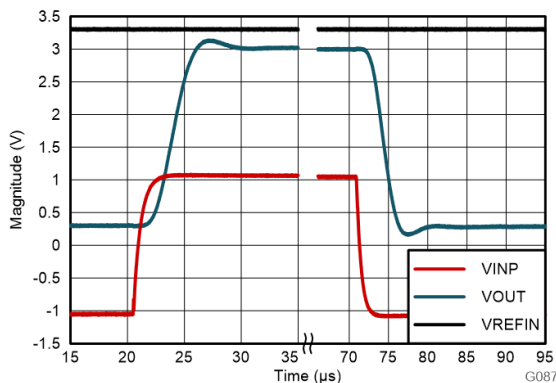
図 8-4. AMC0380R-Q1 のステップ応答
