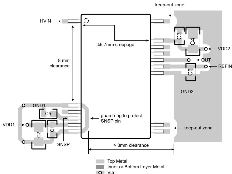
図 8-6. AMC0380R-Q1 の推奨レイアウト
