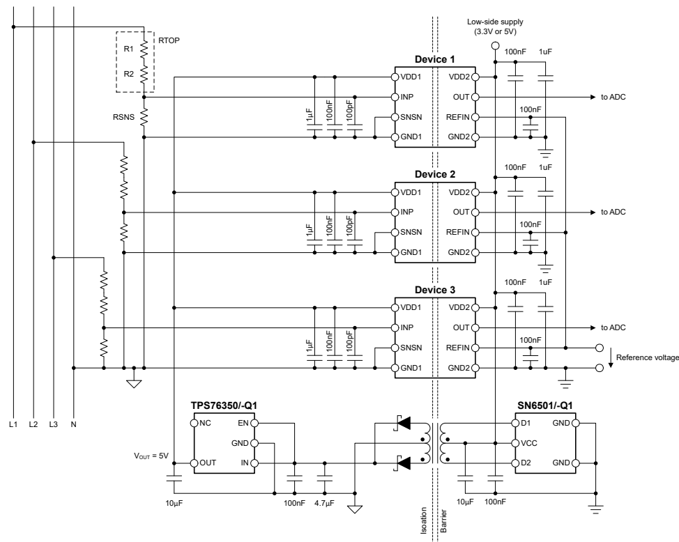
図 8-1. 代表的なアプリケーションで使用 AMC0380R-Q1
