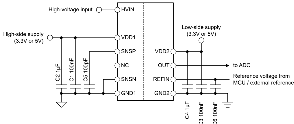
図 8-5. AMC0380R-Q1 のデカップリング
