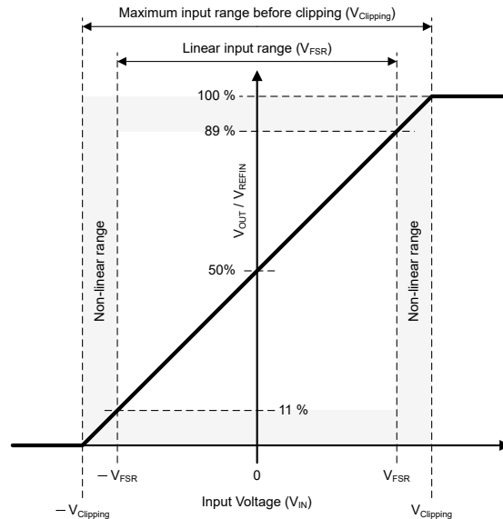
図 7-2. AMC0380R-Q1 の入力から出力への伝達曲線
