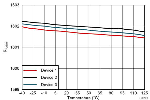
図 6-8. 分圧比と温度との関係
