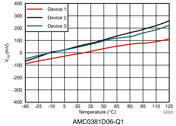
図 6-14. 入力オフセット電圧と温度との関係
