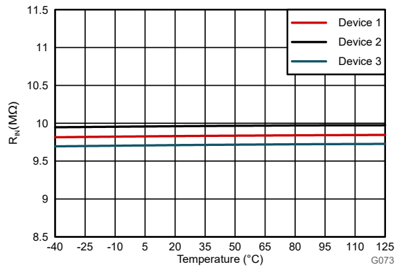
図 6-5. 入力抵抗と温度との関係
