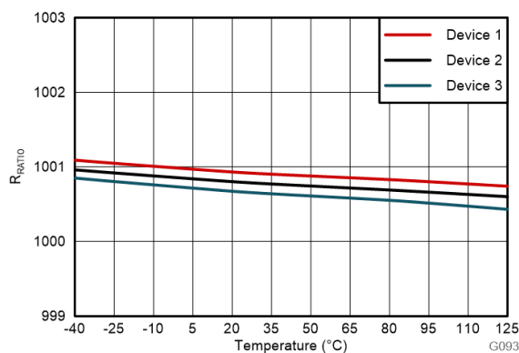
図 6-7. 入力抵抗と温度との関係
