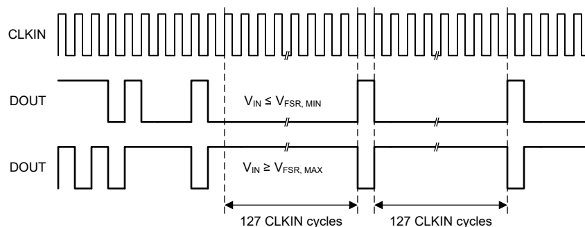
図 7-5. AMC0386-Q1 のフルスケール出力
