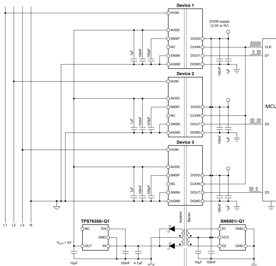
図 8-1. 代表的なアプリケーションで使用 AMC0386-Q1
