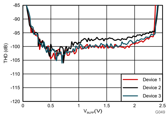
図 6-30. 全高調波歪みと入力信号振幅との関係
