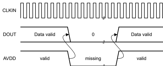
図 7-6. ハイサイド電源が消失した場合の AMC0386-Q1 の出力
