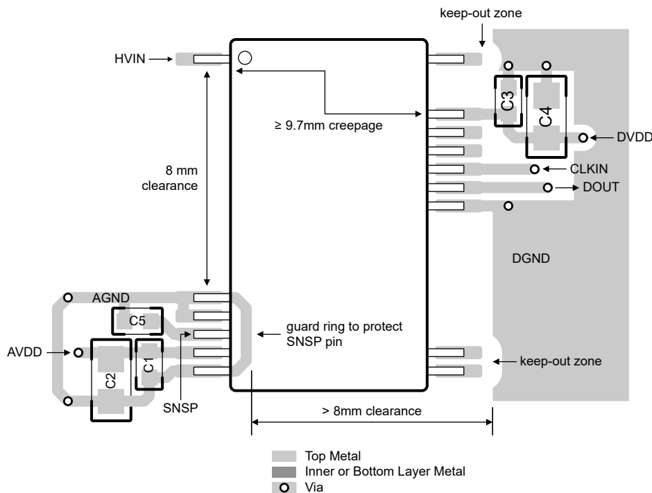
図 8-5. AMC0386-Q1 の推奨レイアウト
