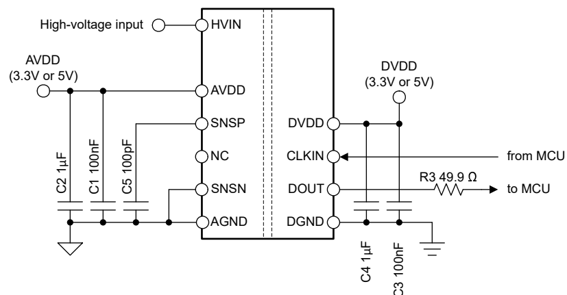
図 8-4. AMC0386-Q1 のデカップリング
