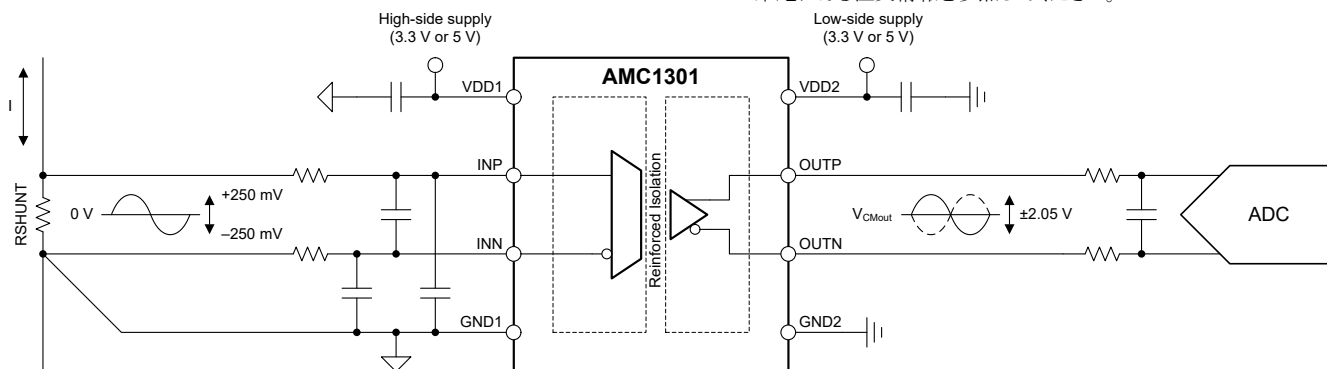
簡略回路図
