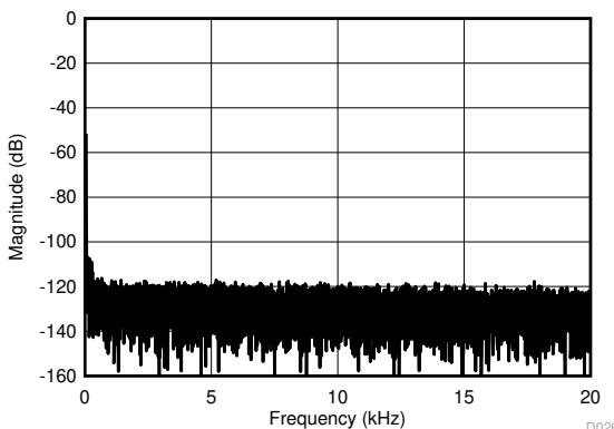
図 6-32. 35Hz 入力信号に対する周波数スペクトラム
