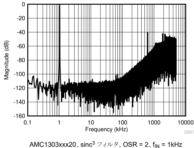
図 7-1. 量子化ノイズ成形
