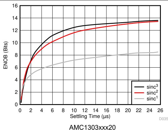
図 8-4. 測定された実効ビット数とセトリング時間との関係
