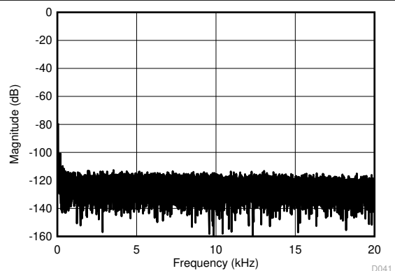
図 6-31. 35Hz 入力信号に対する周波数スペクトラム
