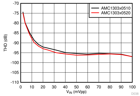
図 6-25. 全高調波歪みと入力信号振幅との関係
