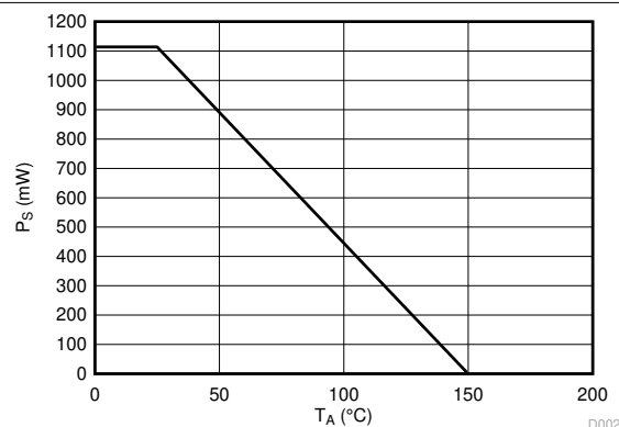
図 6-4. VDE に従う安全性制限電力の熱特性低下曲線
