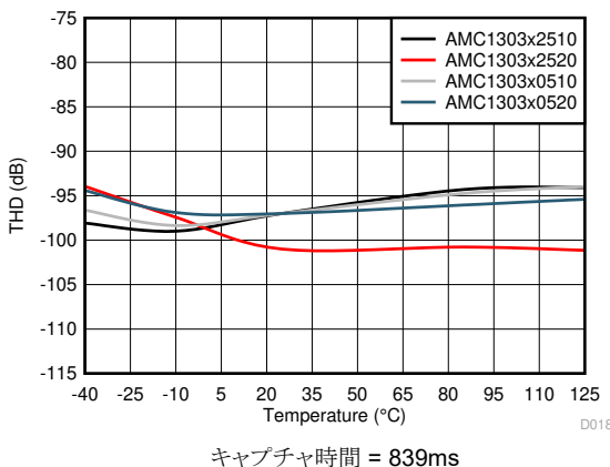
図 6-22. 全高調波歪みと温度との関係
