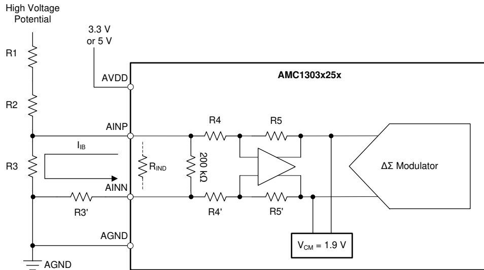
図 8-6. AMC1303x25x を絶縁電圧検出に使用する方法
