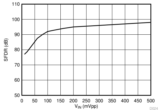
図 6-29. スプリアスフリー ダイナミック レンジと入力信号振幅との関係
