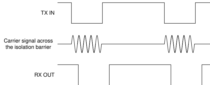
図 7-4. OOK ベースの変調方式
