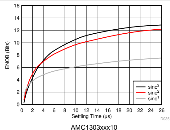
図 8-5. 測定された実効ビット数とセトリング時間との関係
