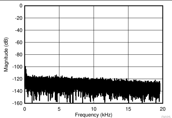
図 6-33. 35Hz 入力信号に対する周波数スペクトラム
