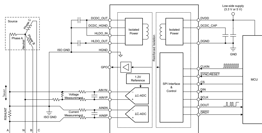
エネルギー・メーターにおける AMC130M02 の代表的なアプリケーション
