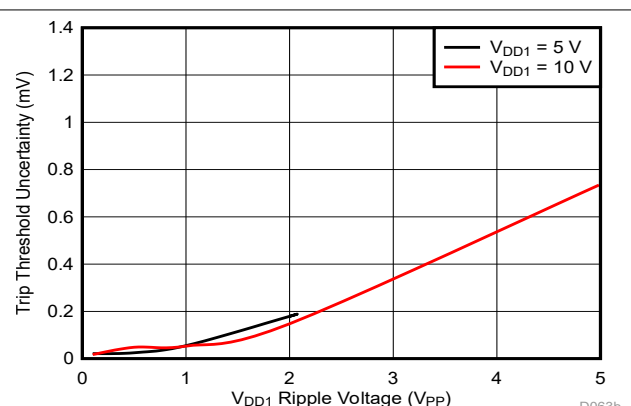
図 7-5. VDD1 リップル電圧に対するトリップスレッショルド感度 (Cmp1、 f_{\text{RIPPLE}} = 10\text{kHz} )
