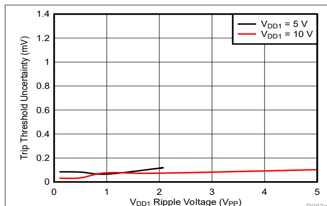
図 7-4. VDD1 リップル電圧に対するトリップスレッショルド感度 (Cmp0、 f_{\text{RIPPLE}} = 10\text{kHz} )
