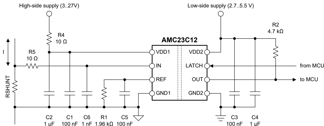
図 7-6. AMC23C12 のデカップリング
