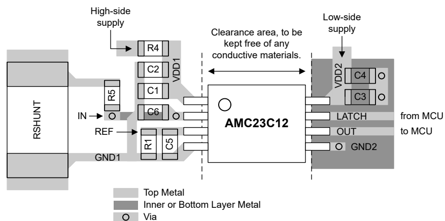
図 7-7. AMC23C12 の推奨レイアウト
