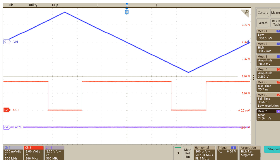
図 7-3. 三角入力波に対する AMC23C12 の出力応答
