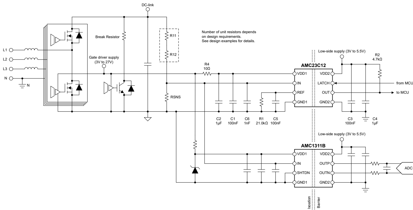
図 7-2. AMC23C12 による過電圧検出
