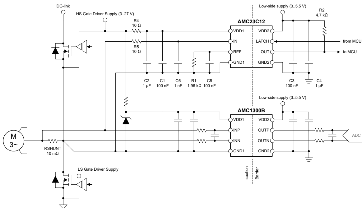
図 7-1. AMC23C12 による過電流の検出
