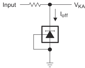
图 6-3. Test Circuit for I_{off}
