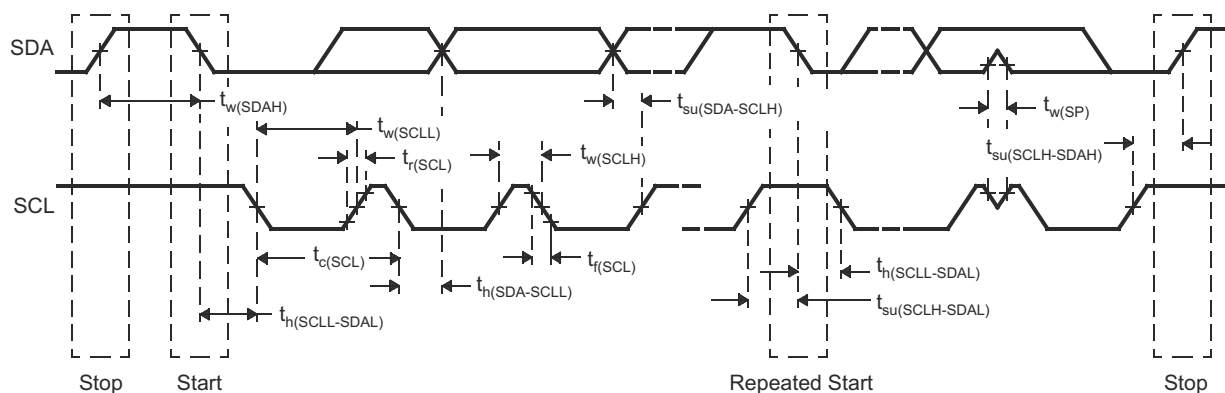
図 7-14. I2C タイミング図
