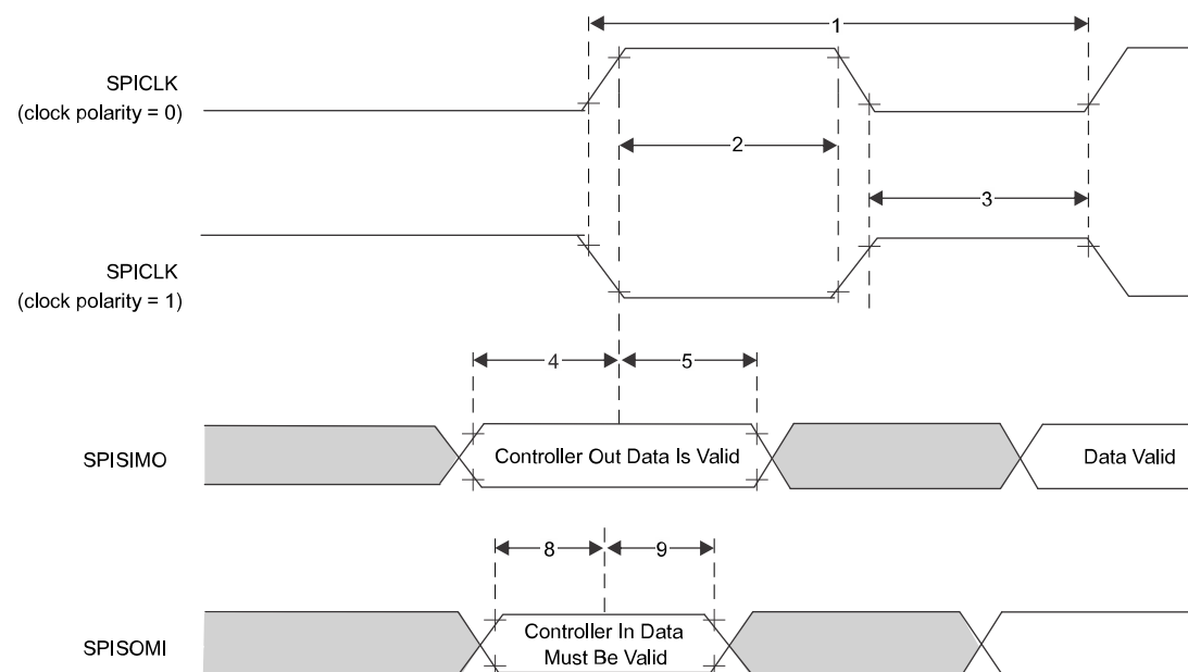
図 7-7. SPI コントローラ モードの外部タイミング (クロック位相 = 1)
