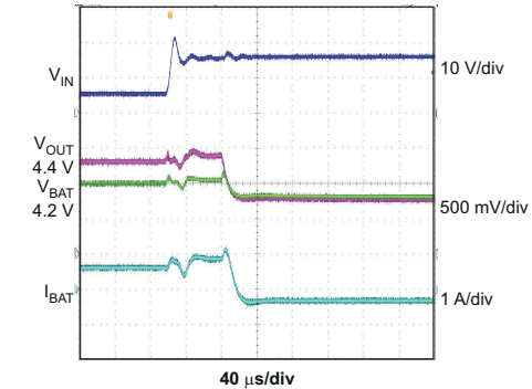
图 10-9. OVP Fault
