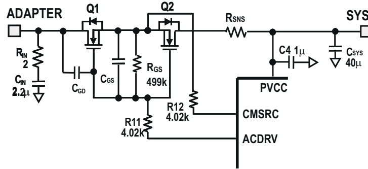
图 10-3. Input ACFET and RBFET
