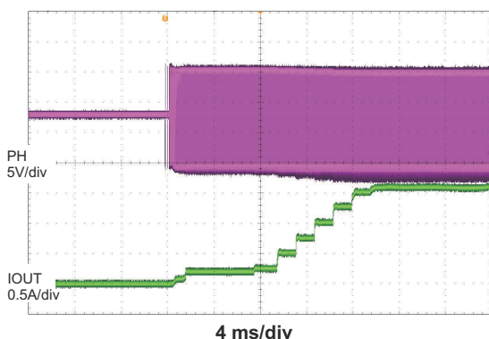
図 8-3. Current Soft Start
