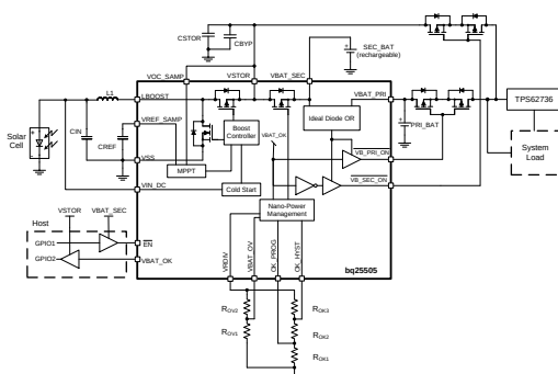
概略回路図
