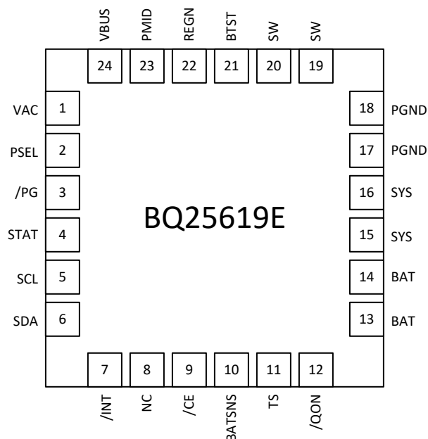
図 6-2. BQ25619E RTW Package 24-Pin WQFN Top View
