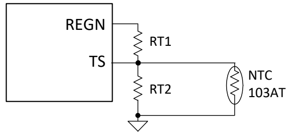
図 8-4. TS Pin Resistor Network
