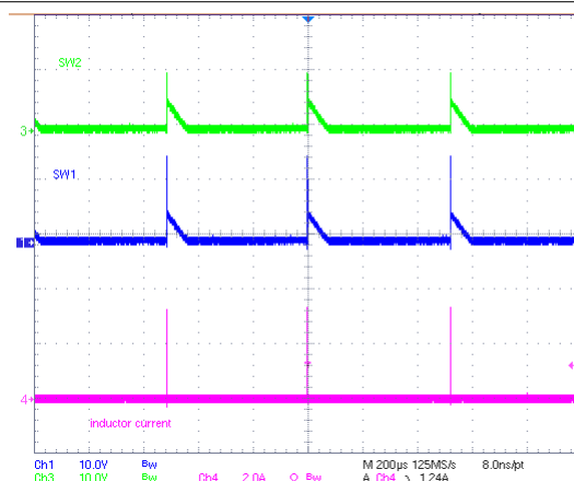
图 9-4. Buck Mode PFM without OOA
