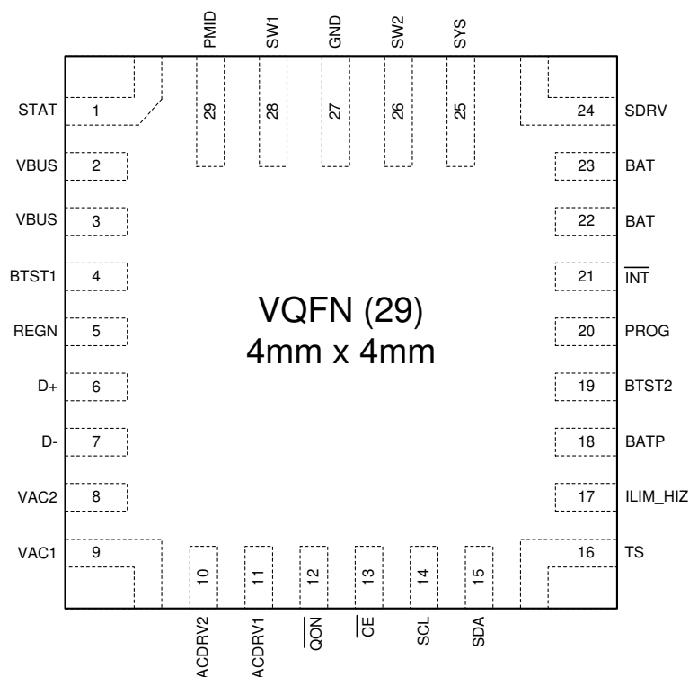
图 6-1. RQM Package 29-Pin VQFN Top View
