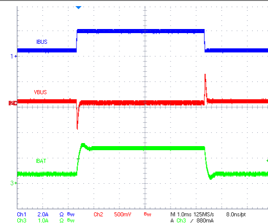
图 9-6. OTG Startup at 500-mA Load
