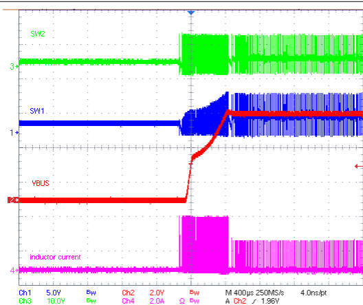
图 9-3. Buck Mode PFM with OOA
