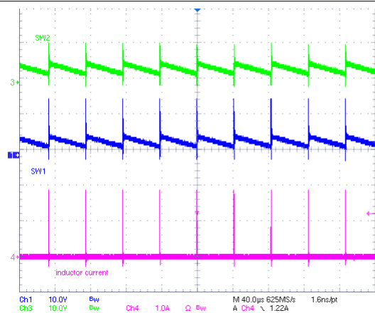
图 9-3. Buck Mode PFM with OOA
