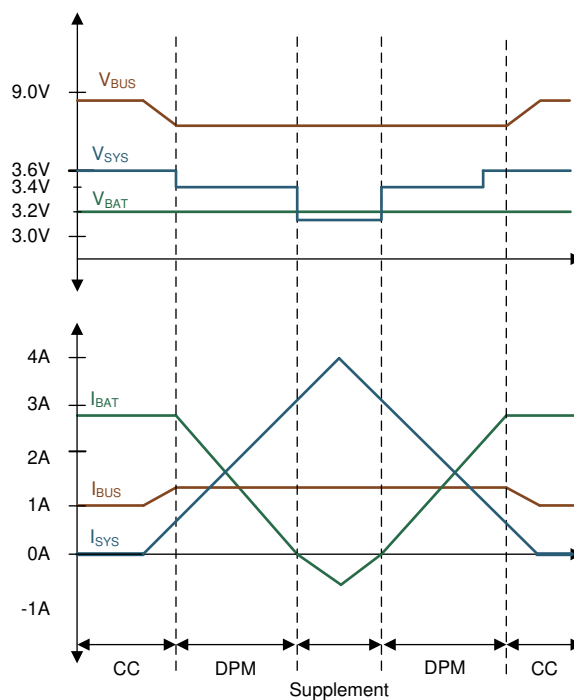
图 8-9. DPM Response
