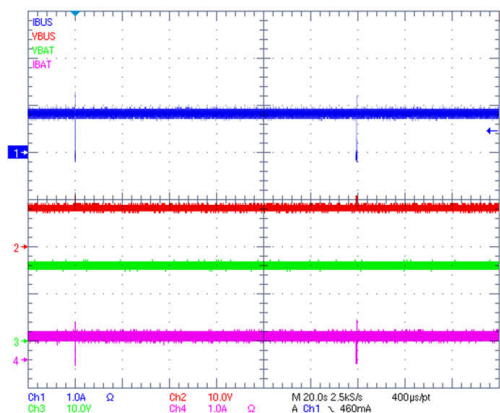
図 9-9. MPPT Operation
