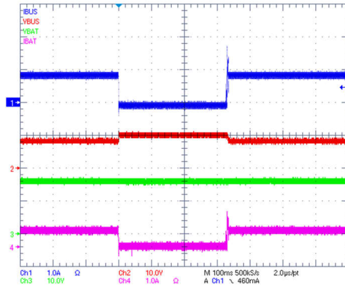
図 9-10. MPPT Operation Zoom
