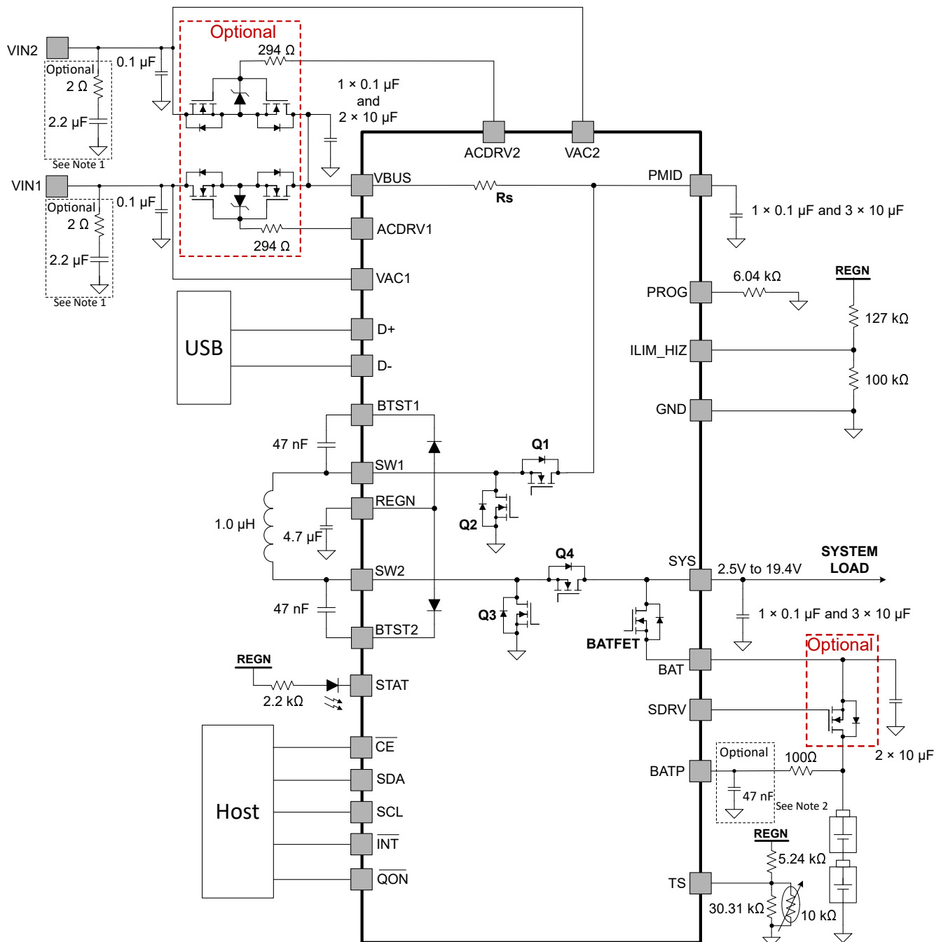
图 9-1. BQ25672 应用图带有两个输入源和 Ship FET
