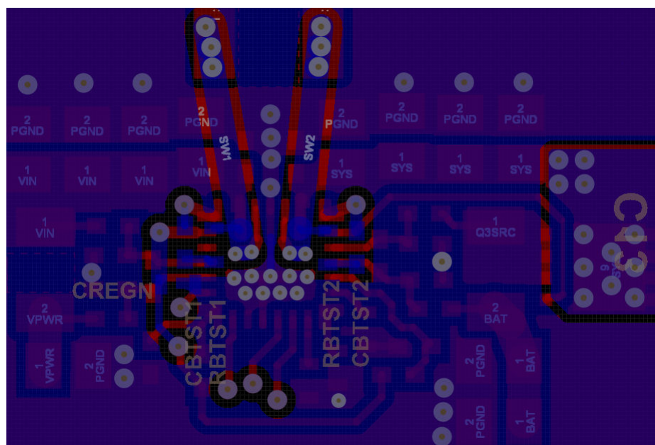
図 8-25. 2 層 PCB レイアウト例の最下層では、青/紫の部分が GND
