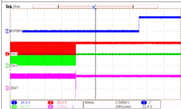
図 8-8. バッテリー プラグイン検出
