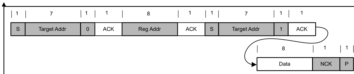
図 6-17. 単発読み取り
