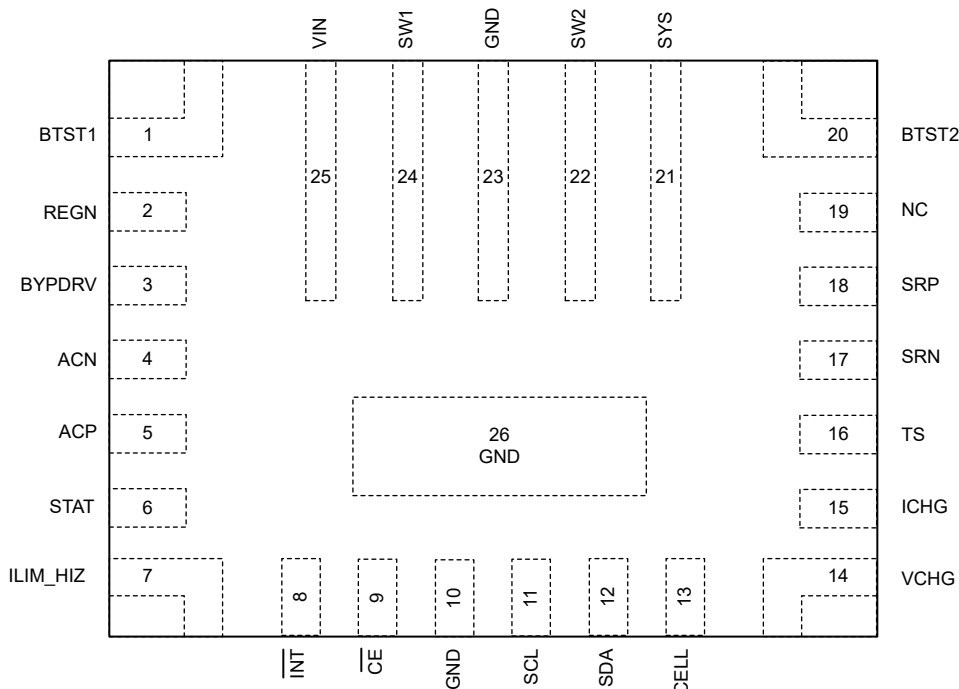
図 4-1. BQ25692-Q1 RBA パッケージ ウェットابل フランク付き 26 ピン WQFN-HR (上面図)
