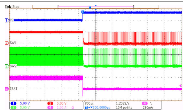
図 8-5. CE ピンで充電を有効化
