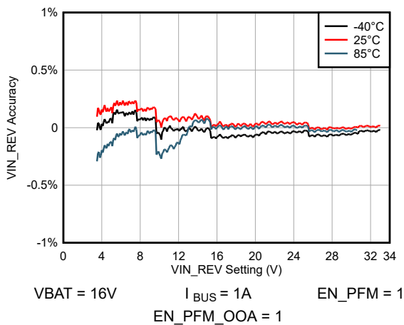
図 5-15. VIN_REV の精度
