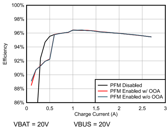
図 5-9. PWM/PFM/OOA 各モード別 5S の充電効率対充電電流特性
