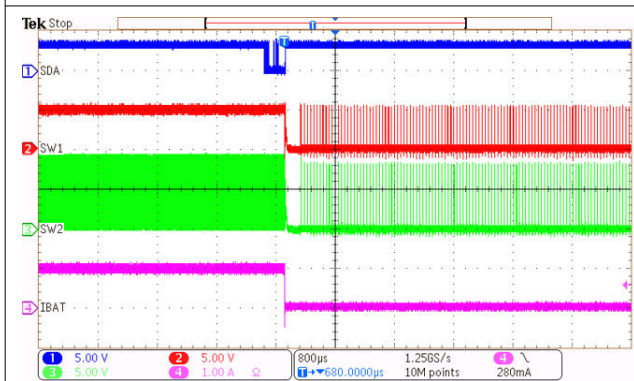
図 8-4. I 2 C で充電を有効化
