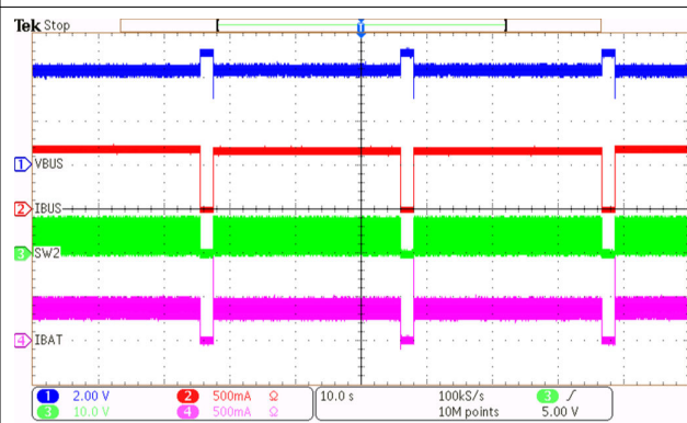
図 8-15. OOA なしでの順方向昇圧モード PFM
