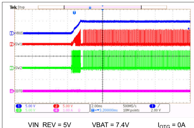
図 8-20. OTG 負荷なしで逆方向モードを有効化
