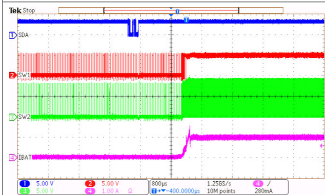
図 8-2. 充電が有効な状態でアダプタ プラグイン
