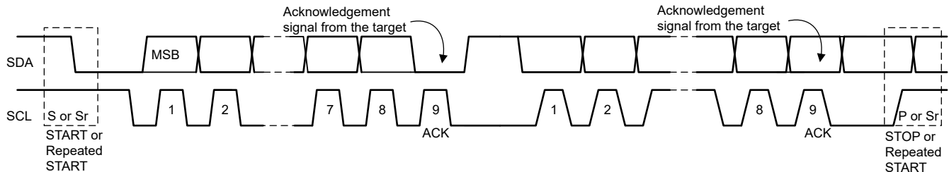
図 6-14. I 2 C バスでのデータ転送
