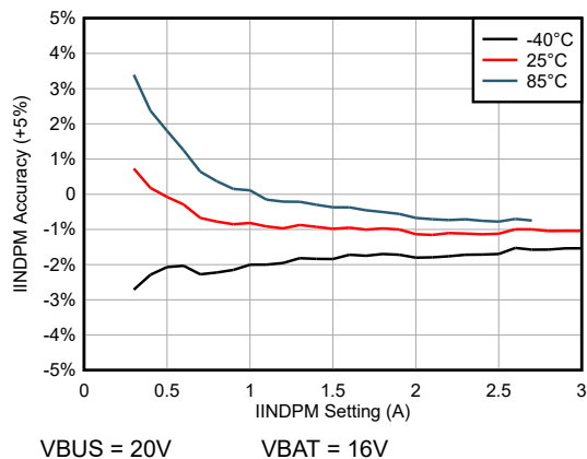
図 5-13. IINDPM の精度
