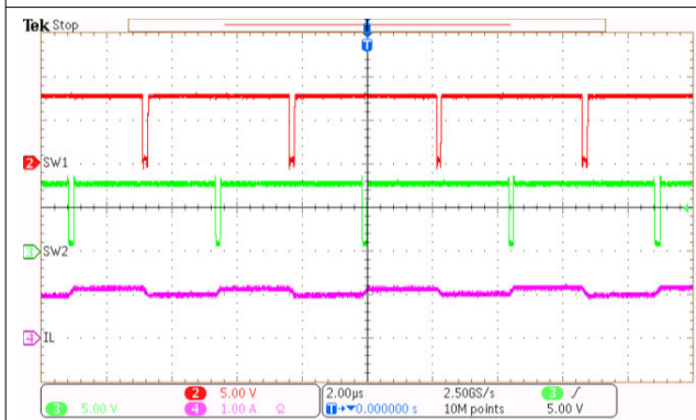
図 8-10. 昇降圧から内部バイパスへの外部バイパス遷移
