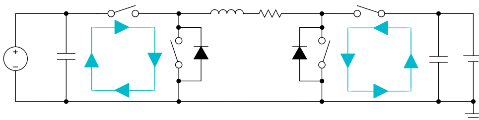
図 8-23. コンバータの高周波電流パス
