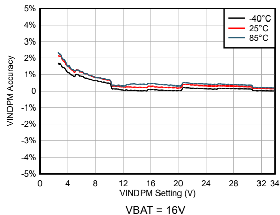
図 5-14. VINDPM の精度
