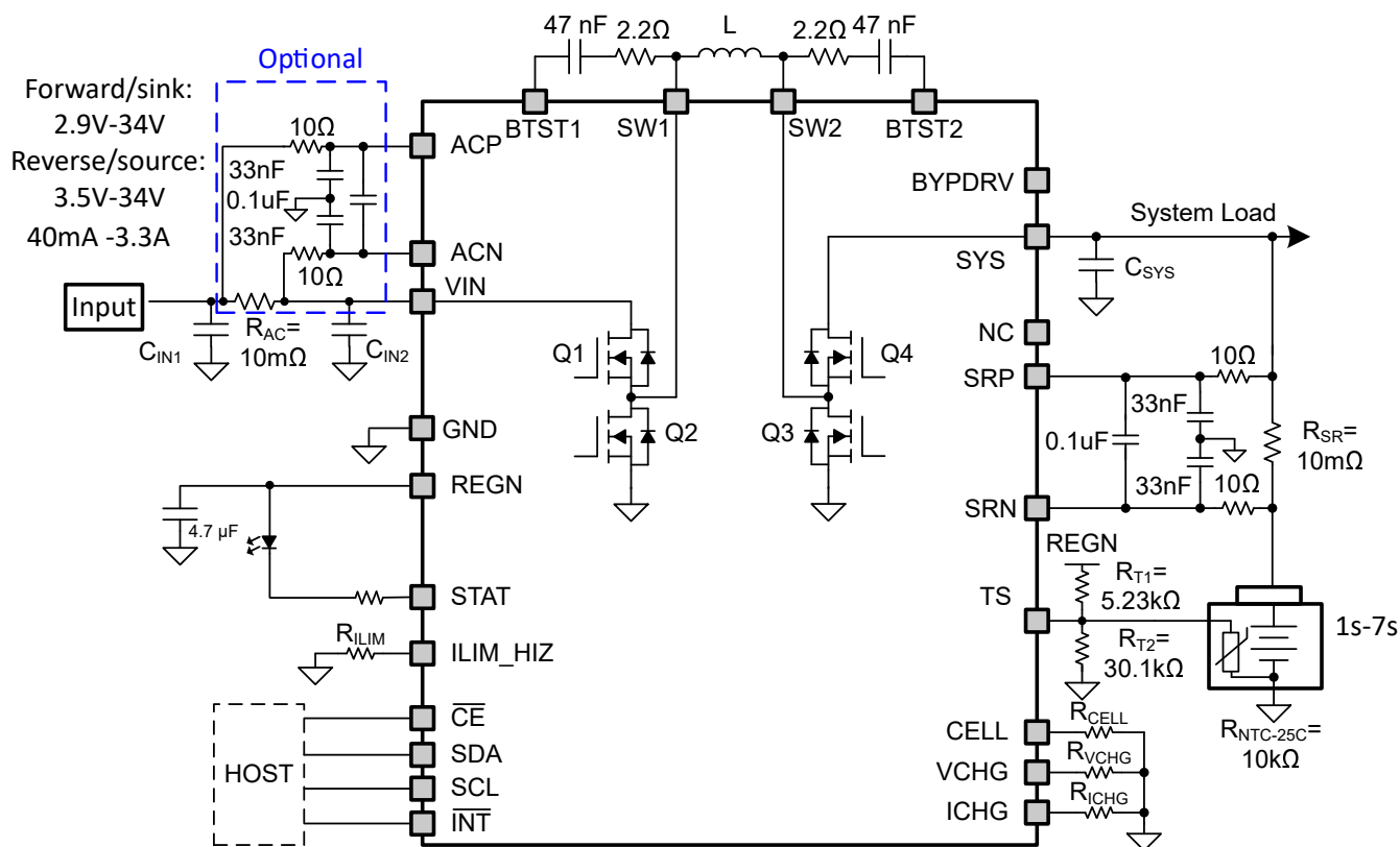
図 8-1. BQ25692-Q1 代表的なアプリケーションの図
