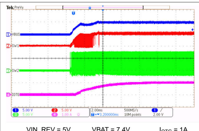
図 8-21. 1A OTG 負荷で逆方向モードを有効化
