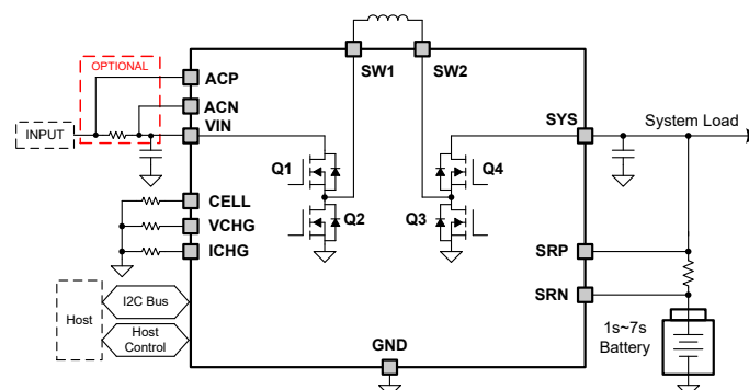
概略回路図
