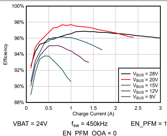
図 5-3. 6S の充電効率対充電電流特性
