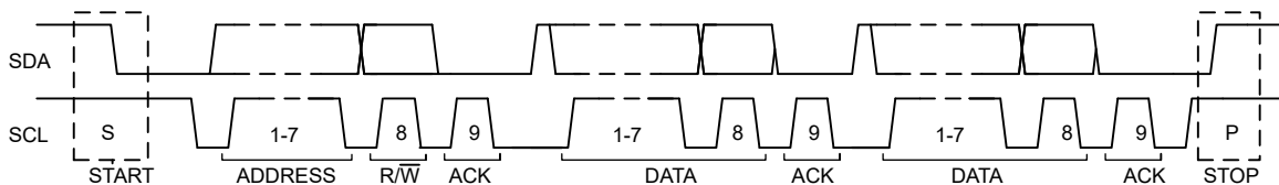
図 6-15. I 2 C バスでのビット転送の完了
