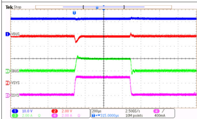
図 8-14. OOA での順方向昇圧モード PFM
