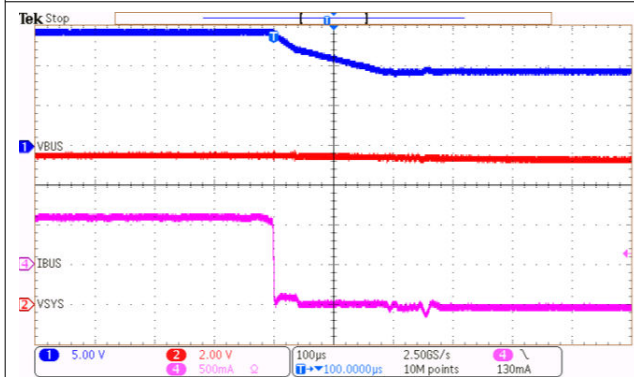
図 8-16. 順方向モード I_{SYS} 過渡応答
