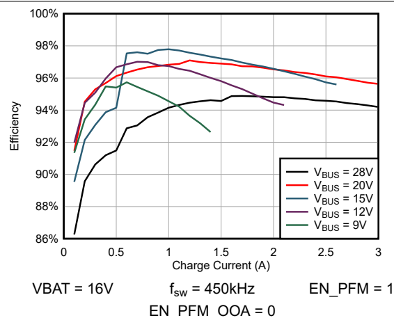
図 5-2. 4S の充電効率対充電電流特性
