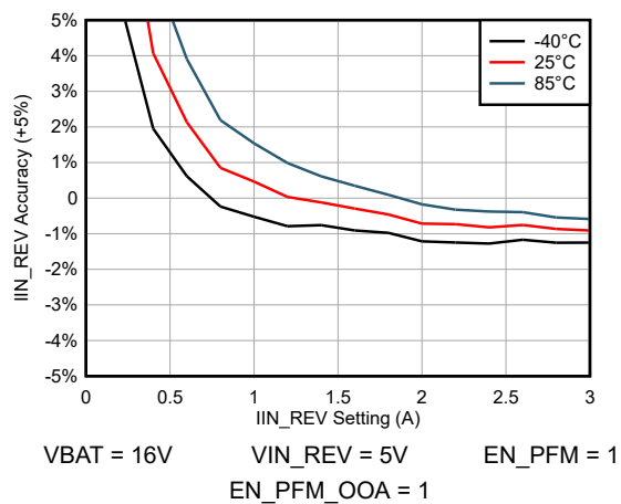
図 5-16. IIN_REV の精度
