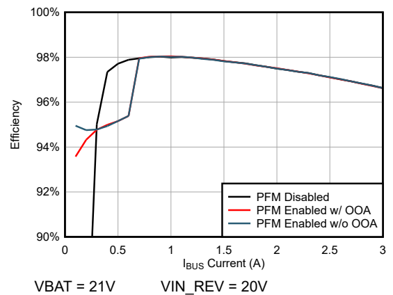
図 5-10. PWM/ PFM/ OOA 各モード別 5S バッテリの OTG 効率対充電電流特性
