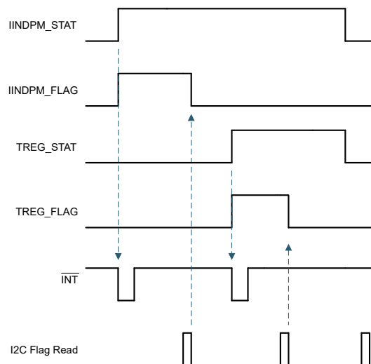
図 6-11. \overline{\text{INT}} 生成の動作の例
