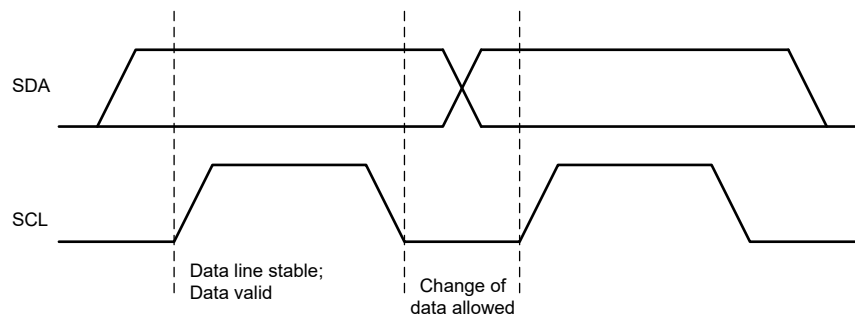
図 6-12. I^2C バスでのビット転送
