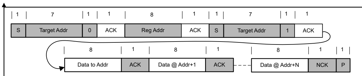
図 6-19. マルチ読み取り
