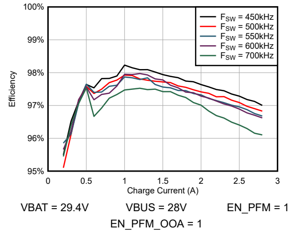
図 5-8. スイッチング周波数別 7S の充電効率対充電電流特性
