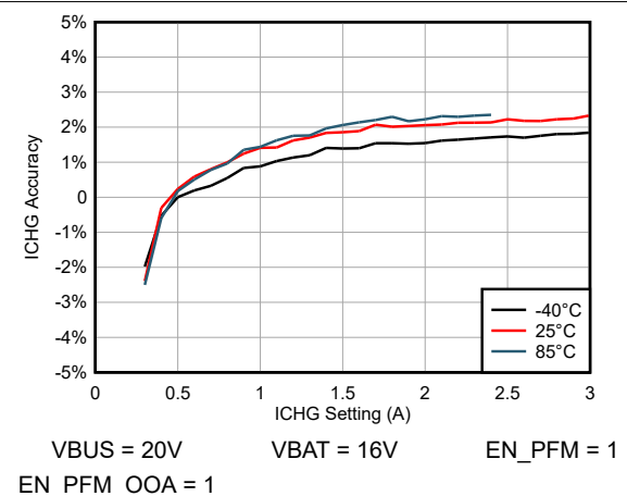
図 5-12. 充電電流精度
