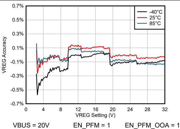
図 5-11. 充電電圧精度
