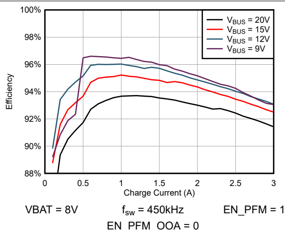
図 5-1. 2S の充電効率対充電電流特性
