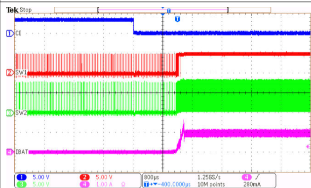
図 8-3. 充電が有効な状態でアダプタ プラグ解除
