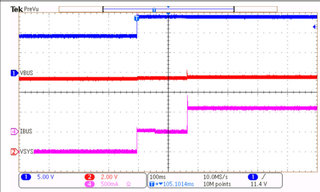
図 8-17. 低 VIN での MPPT レギュレーション
