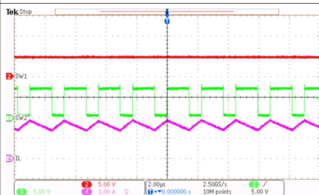
図 8-11. 順方向降圧モード CCM
