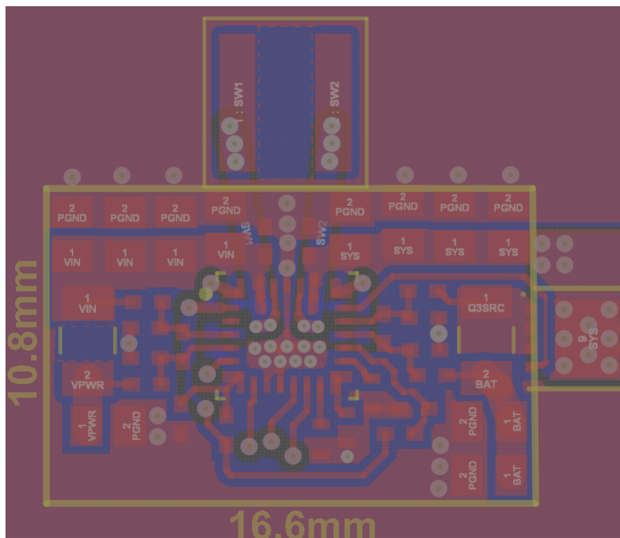
図 8-24. 2層 PCB レイアウト例の最上層 - 赤はグランド
