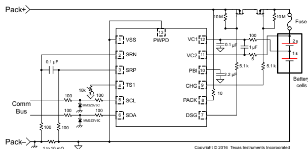
概略回路図
