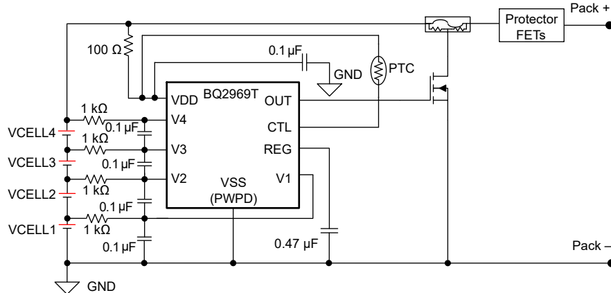
図 8-8. BQ2969T PTC 構成のリファレンス回路図
