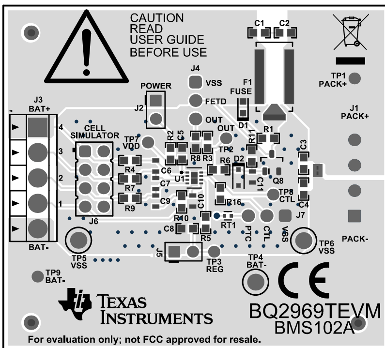
図 8-11. BQ2969T の 2 層基板レイアウト - 上層
