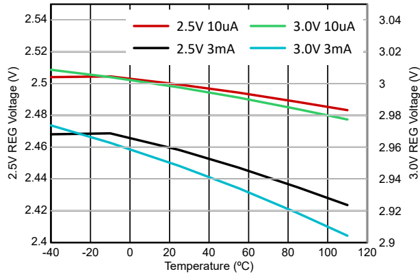
図 6-7. レギュレータ出力と温度との関係 (2.5V および 3V 設定)
