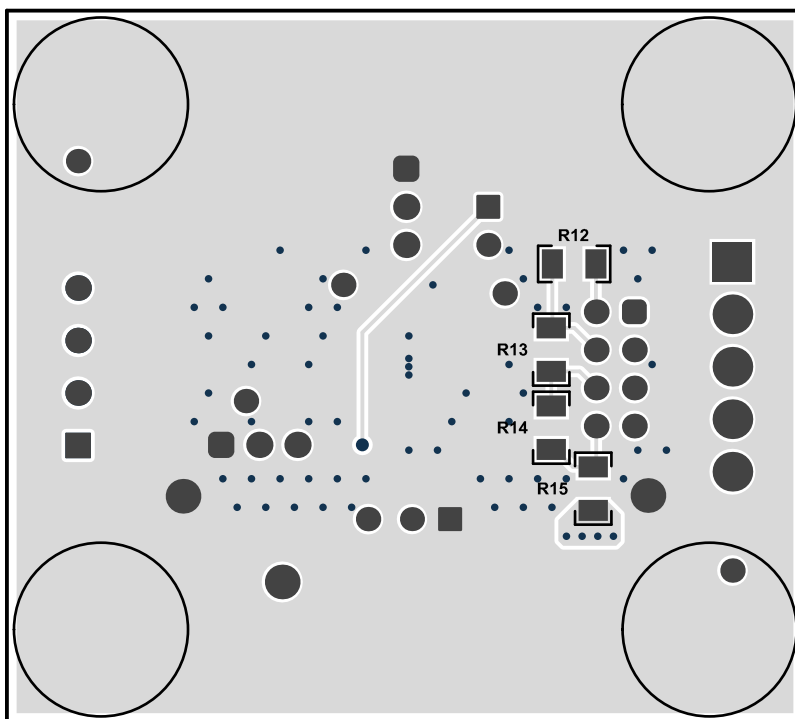
図 8-12. BQ2969T の 2 層基板レイアウト - 下層
