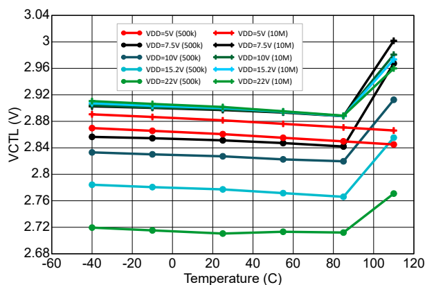
図 6-11. CTL 電圧スレッシュホールドの精度 ( V_{CTL} ) と温度との関係
