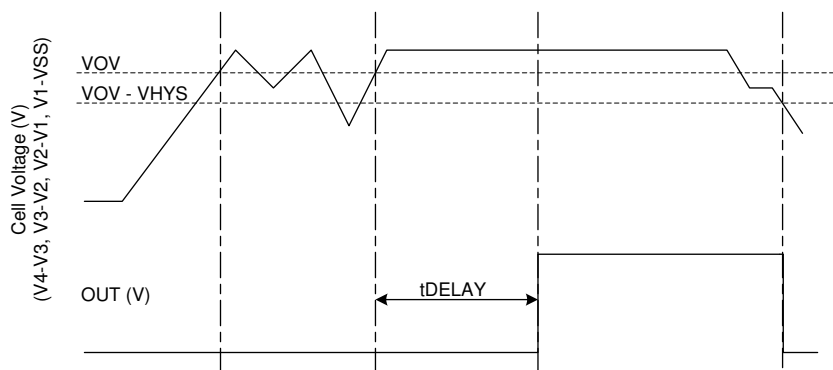
図 7-2. OUT の過電圧検知のタイミング
