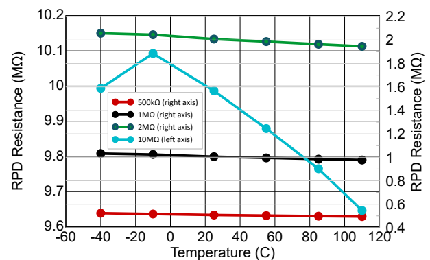
図 6-12. CTL プルダウン抵抗 ( R_{PD} ) と温度との関係
