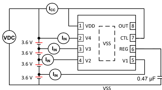
図 7-5. IC 消費電流テストの構成
