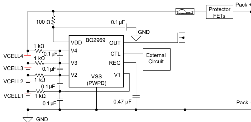
図 8-1. BQ2969T 4 直列セルの代表的な実装 (概略回路図)
