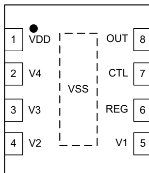
図 5-1. 2 ～ 4 直列の BQ2969T (上面図)
