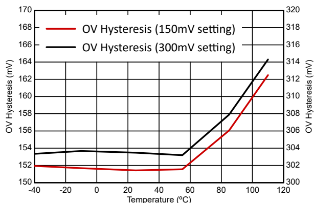
図 6-2. 過電圧ヒステリシス ( V_{OVHYS} ) と温度との関係
