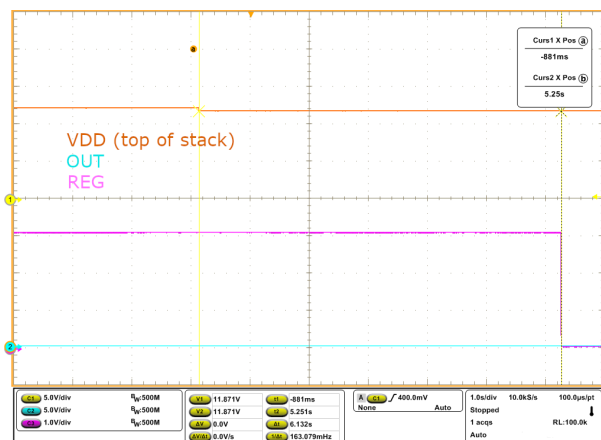
図 8-6. レギュレータを無効化する低電圧検出
