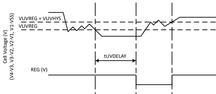
図 7-3. REG 出力のタイミング
