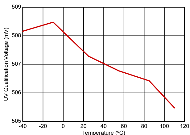
図 6-4. 低電圧認定電圧 ( V_{UVQUAL} ) と温度との関係
