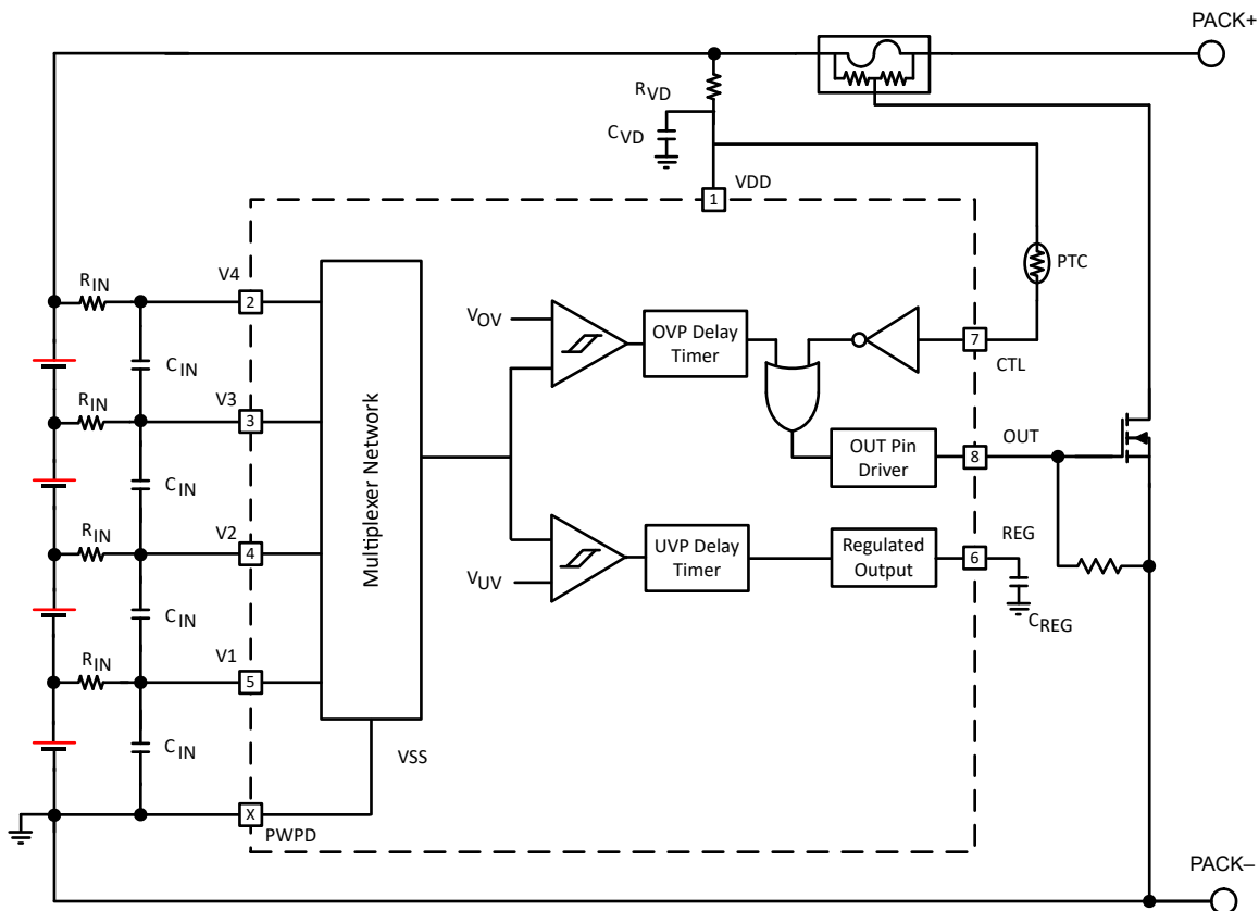
図 7-1. BQ2969T のブロック図
