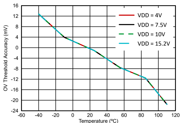
図 6-1. 過電圧スレッシュホールドの精度 ( V_{OA} ) と温度との関係
