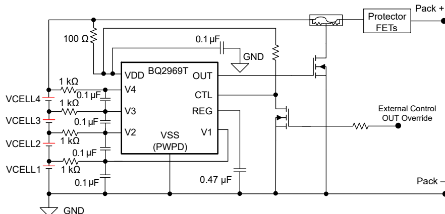
図 8-10. BQ2969T 外部出力オーバードライブ構成のリファレンス回路図
