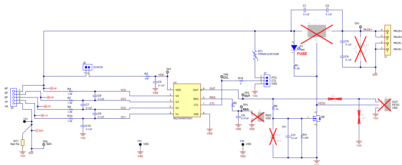
図 8-2. BQ2969T 4 直列セル回路図 - プロテクタおよびヒューズ解除回路
