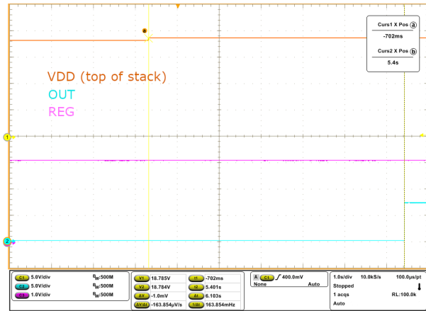
図 8-4. 過電圧保護トリガ
