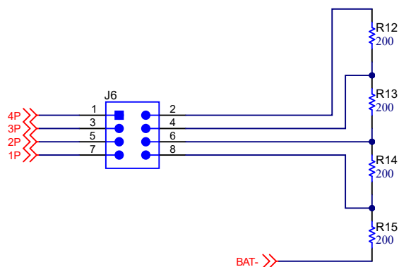
図 8-3. BQ2969T 4 直列セル回路図 - セル シミュレータ回路
