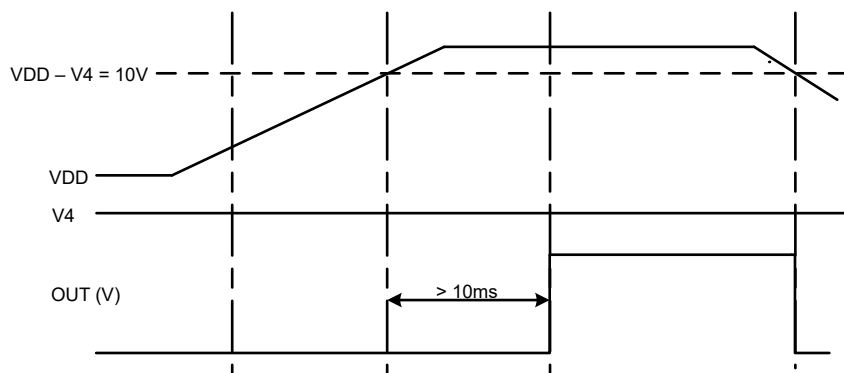
図 7-4. カスタマー テスト モードのタイミング
