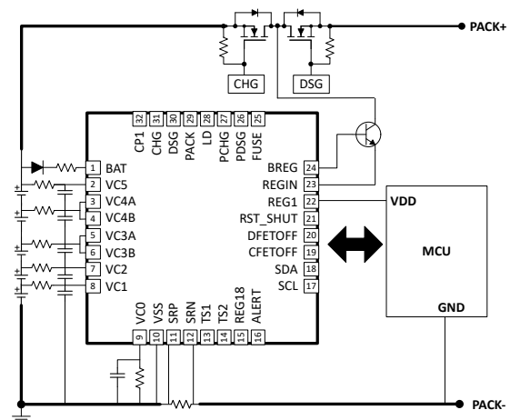
概略回路図
