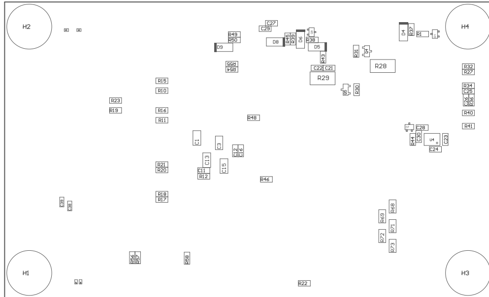
図 10-8. BQ76922EVM Bottom Assembly
