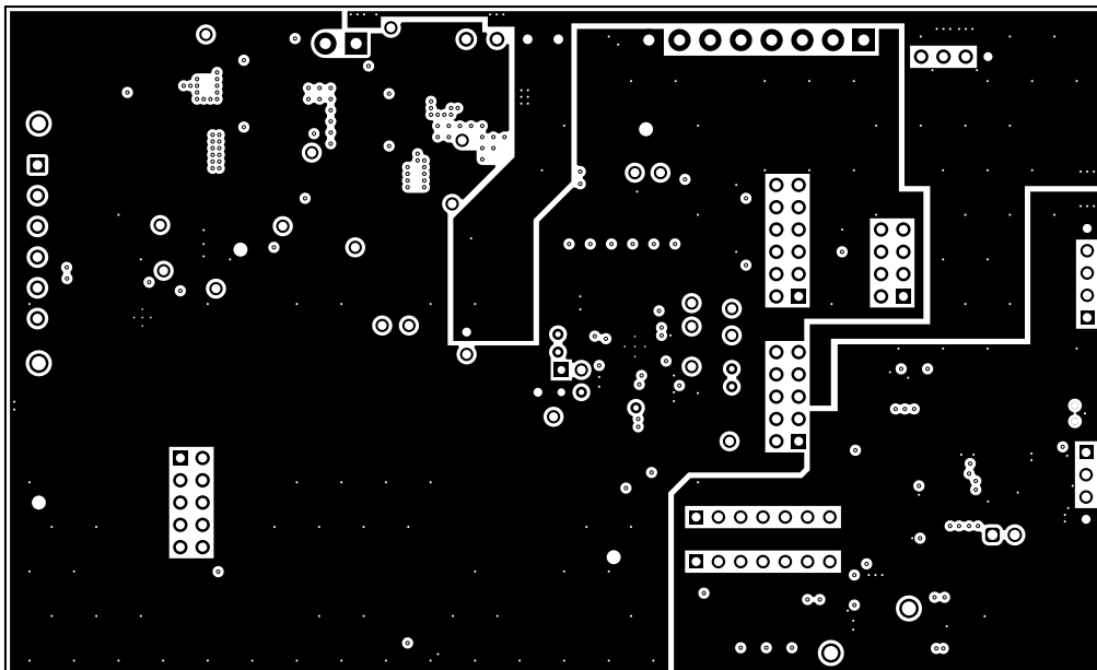
図 10-4. BQ76922EVM Layer 2
