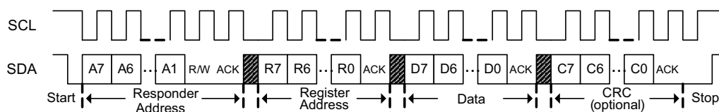
図 7-6. I 2 C Write
