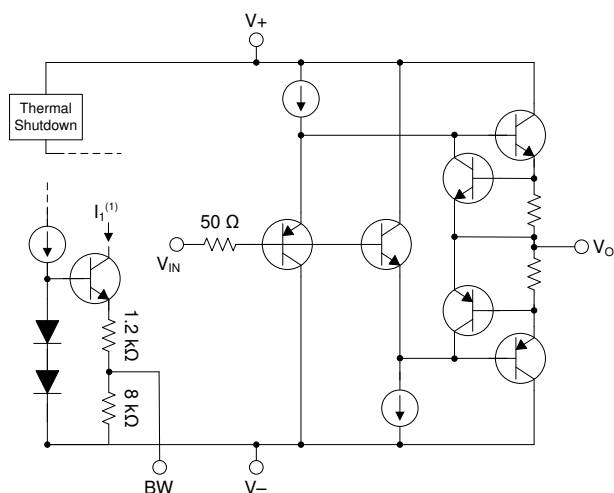
図 7-2. Internal Block Diagram: SOIC
