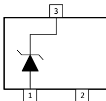
図 5-1. DBZ パッケージ、3 ピン SOT-23 (上面図)
