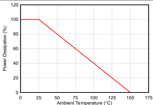
図 6-3. 電力ディレーティング曲線
